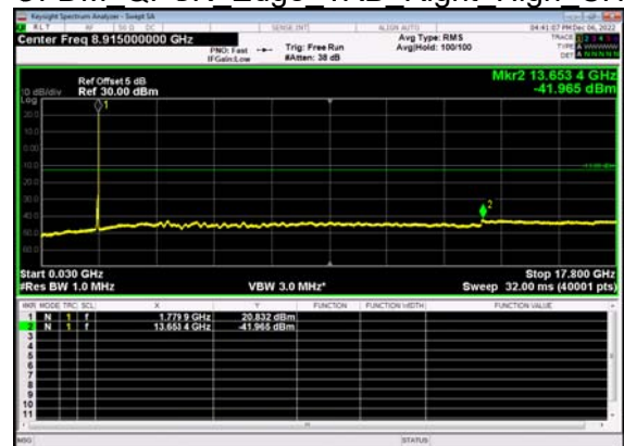
N66(30M)_DFT-s- OFDM QPSK Edge 1RB Right High CH
