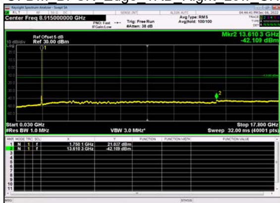
N66(40M)_DFT-s- OFDM BPSK Edge 1RB Right Low CH
