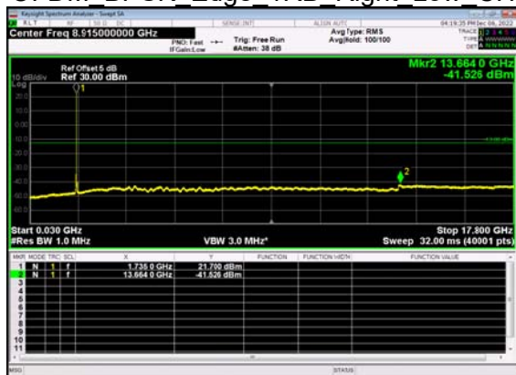
N66(25M)_DFT-s- OFDM BPSK Edge 1RB Right Low CH
