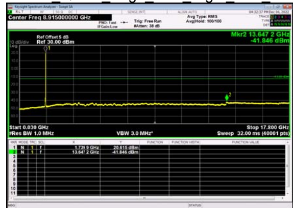
N66(30M)_DFT-s- OFDM QPSK Edge 1RB Right Low CH
