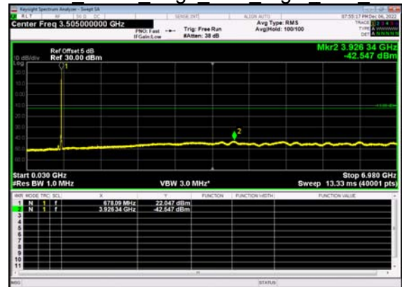
N71(15M)_DFT-s- OFDM BPSK Edge 1RB Right Low CH
