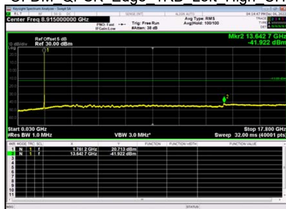
N66(20M)_DFT-s- OFDM QPSK Edge 1RB Left High CH
