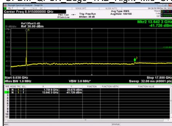
N66(30M)_DFT-s- OFDM QPSK Edge 1RB Right Mid CH
