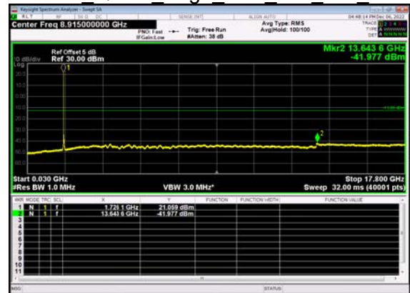
N66(40M)_DFT-s- OFDM QPSK Edge 1RB Left Mid CH
