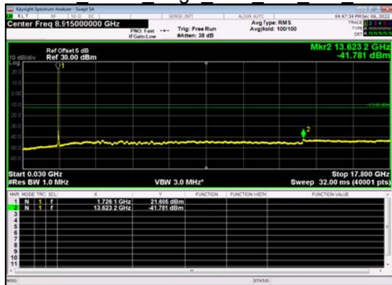
N66(40M)_DFT-s- OFDM BPSK Edge 1RB Left Mid CH
