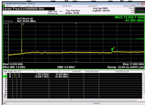
N66(40M)_DFT-s- OFDM BPSK Edge 1RB Left High CH
