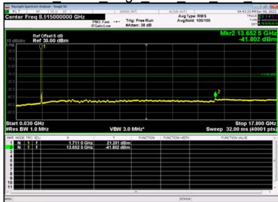
N66(40M)_DFT-s- OFDM BPSK Edge 1RB Left Low CH
