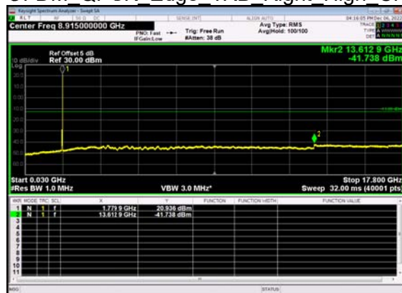
N66(20M)_DFT-s- OFDM QPSK Edge 1RB Right High CH
