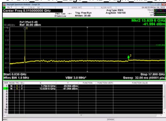
N66(40M)_DFT-s- OFDM BPSK Edge 1RB Right Mid CH
