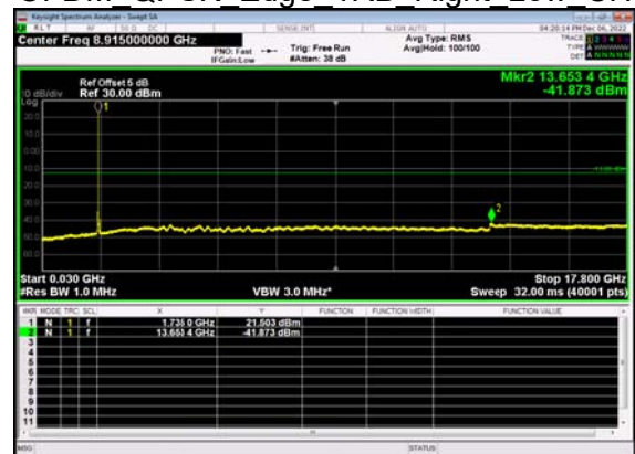
N66(25M)_DFT-s- OFDM QPSK Edge 1RB Right Low CH
