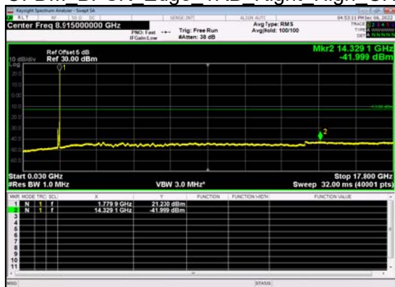
N66(40M)_DFT-s- OFDM BPSK Edge 1RB Right High CH
