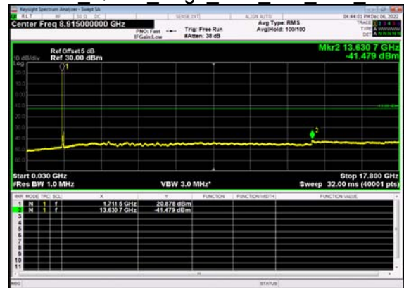
N66(40M)_DFT-s- OFDM QPSK Edge 1RB Left Low CH
