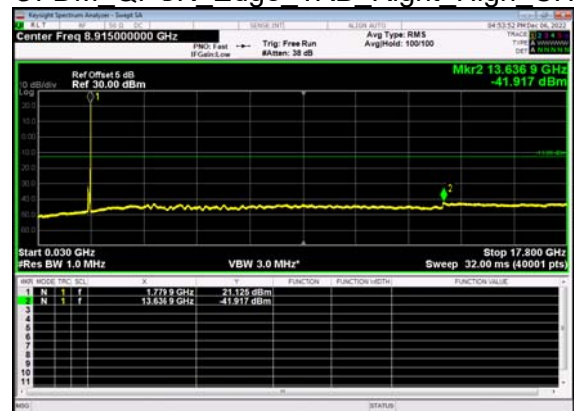
N66(40M)_DFT-s- OFDM QPSK Edge 1RB Right High CH
