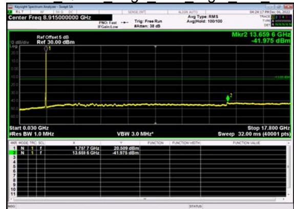
N66(25M)_DFT-s- OFDM QPSK Edge 1RB Right Mid CH
