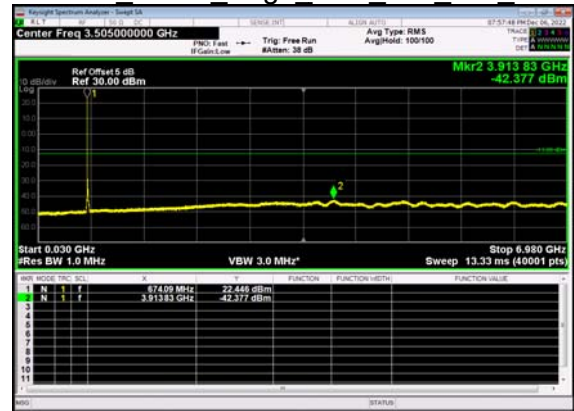
N71(15M)_DFT-s- OFDM BPSK Edge 1RB Left Mid CH
