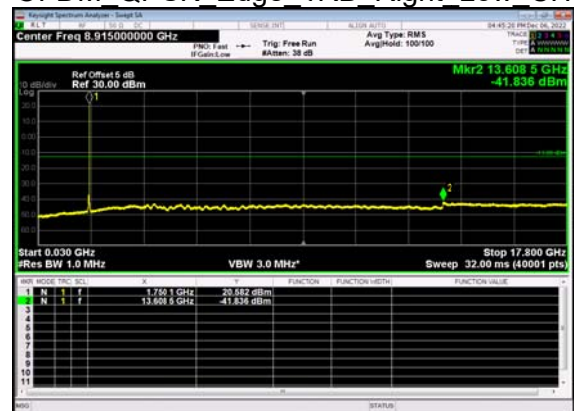
N66(40M)_DFT-s- OFDM QPSK Edge 1RB Right Low CH
