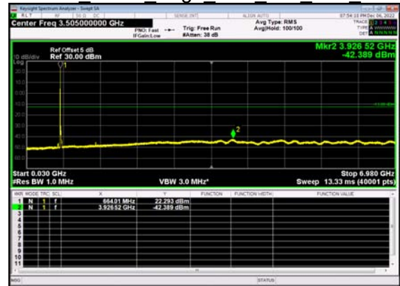
N71(15M)_DFT-s- OFDM BPSK Edge 1RB Left Low CH
