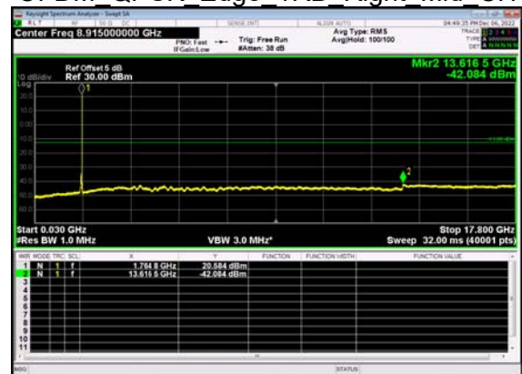
N66(40M)_DFT-s- OFDM QPSK Edge 1RB Right Mid CH
