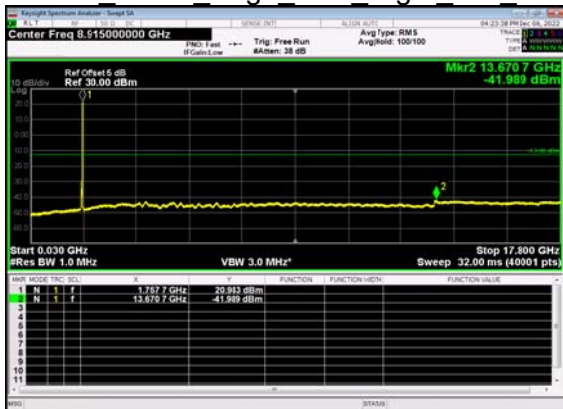
N66(25M)_DFT-s- OFDM BPSK Edge 1RB Right Mid CH
