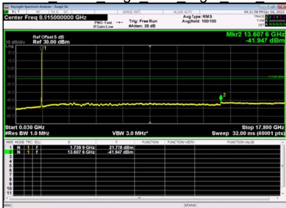
N66(30M)_DFT-s- OFDM BPSK Edge 1RB Right Low CH
