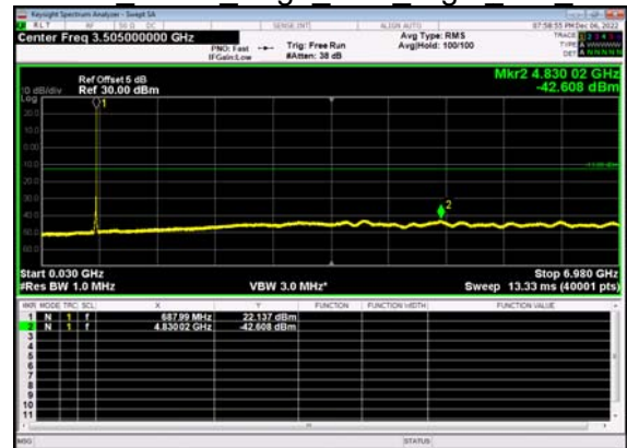
N71(15M)_DFT-s- OFDM BPSK Edge 1RB Right Mid CH
