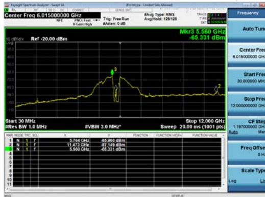
Antenna A
