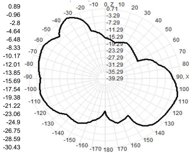
5150.0MHz Total(E1-XZ),Max=0.48dBi
