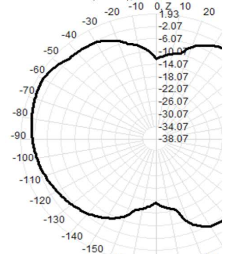
2410.0MHz Total(E2-YZ), Max= 1.84dBi
