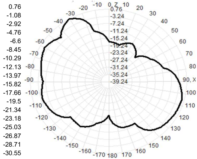
5250.0MHz Total(E1-XZ),Max=0.76dBi
