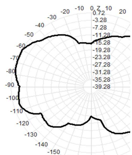
5170.0MHz Total(E2-YZ),Max=0.17dBi
