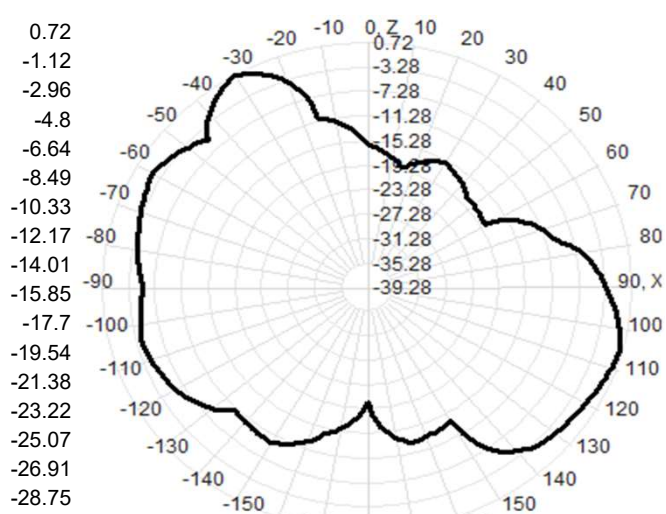
5170.0MHz Total(E1-XZ),Max=0.66dBi
