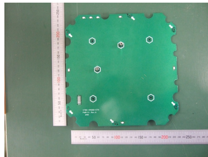
Fig. 26 PCB(2) Side B
