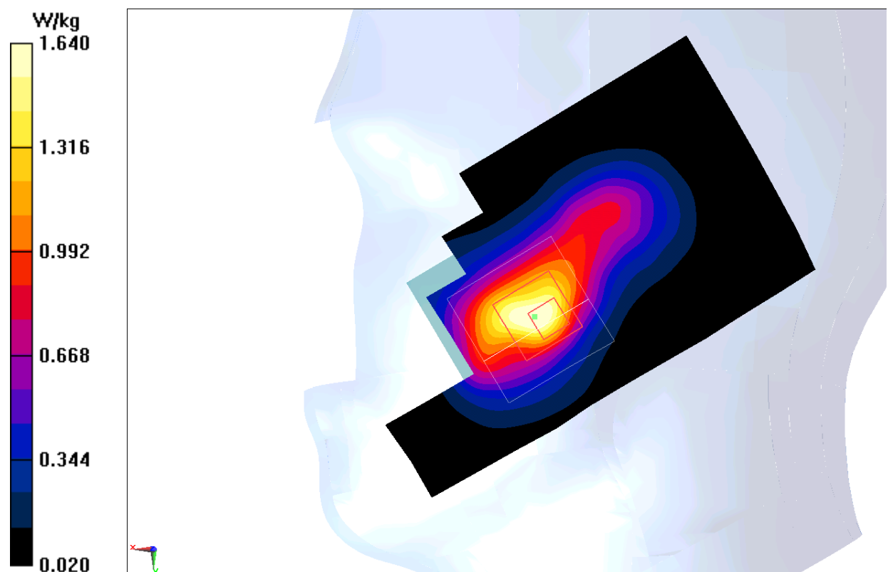
Fig.7 WCDMA1900 CH9538
