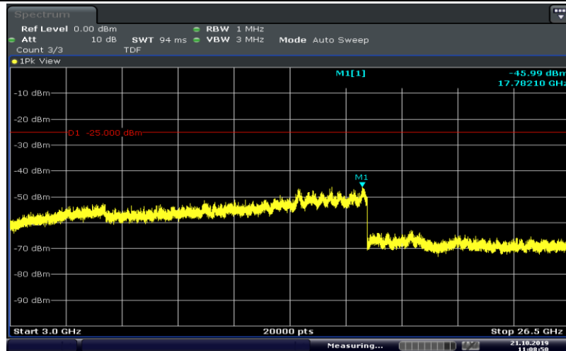
Band38-20MHz-QPSK-37850-100RB#0-Range5:3000~26500MHz
