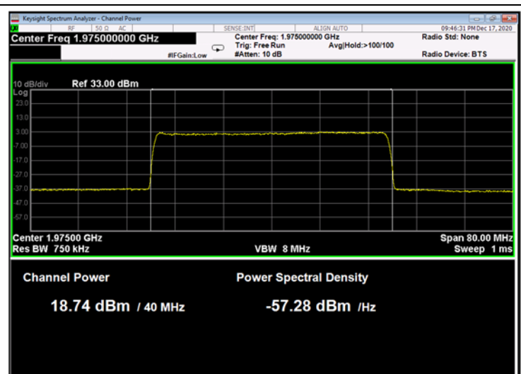
Figure 124: 64QAM 40MHz B.W.; 1975.0MHz, 30kHz
