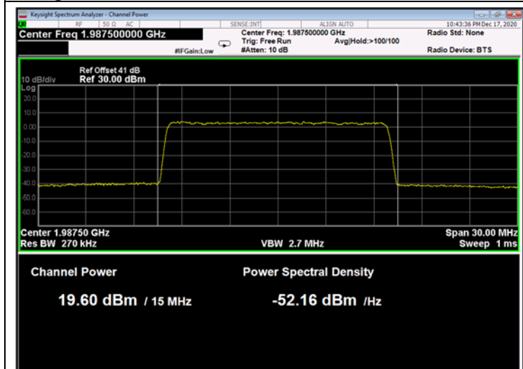
Figure 163: 256QAM 15MHz B.W.; 1987.5MHz, 30kHz
