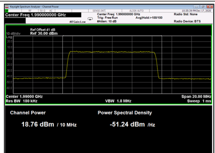
Figure 154: 256QAM 10MHz B.W.; 1990.0MHz, 30kHz
