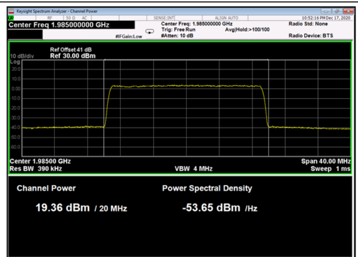
Figure 172: 256QAM 20MHz B.W.; 1985.0MHz, 30kHz
