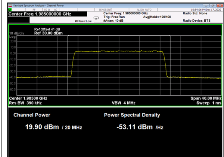
Figure 173: 256QAM 20MHz B.W.; 1985.0MHz, 60kHz
