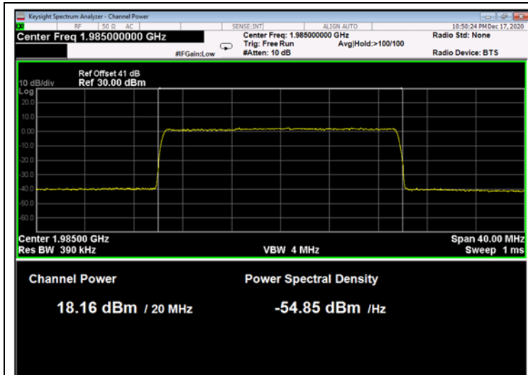
Figure 171: 256QAM 20MHz B.W.; 1985.0MHz, 15kHz
