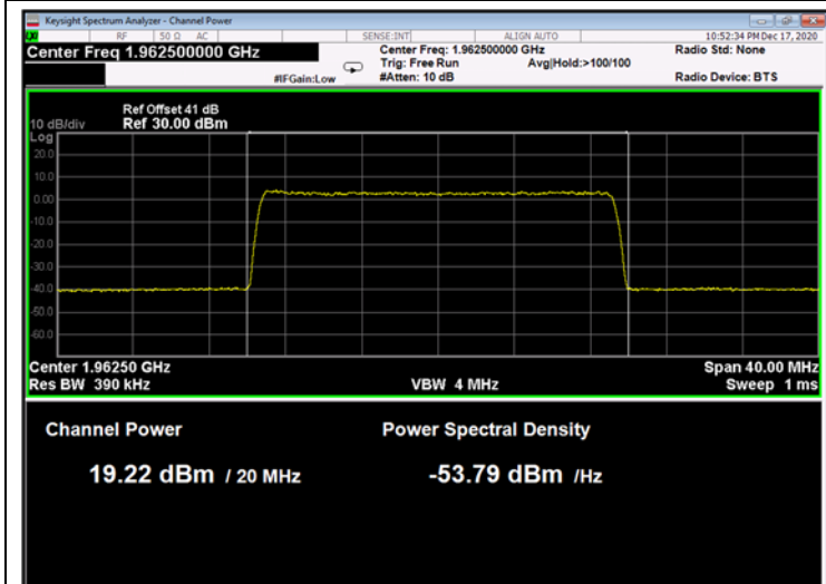
Figure 169: 256QAM 20MHz B.W.; 1962.5MHz, 30kHz
