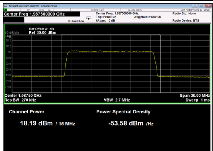
Figure 164: 256QAM 15MHz B.W.; 1987.5MHz, 60kHz
