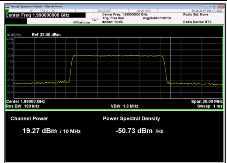
Figure 88: 64QAM 10MHz B.W.; 1990.0MHz, 30kHz
