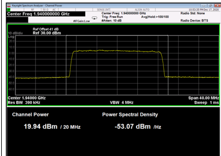
Figure 167: 256QAM 20MHz B.W.; 1940.0MHz, 60kHz
