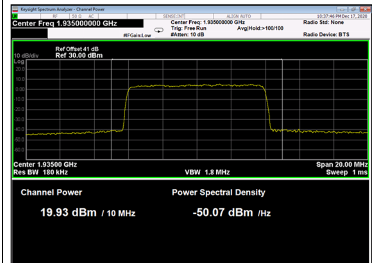
Figure 149: 256QAM 10MHz B.W.; 1935.0MHz, 60kHz
