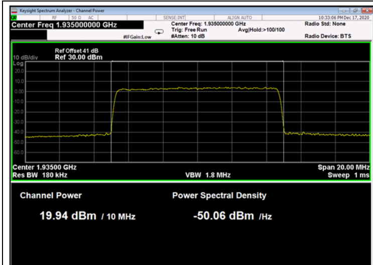
Figure 147: 256QAM 10MHz B.W.; 1935.0MHz, 15kHz
