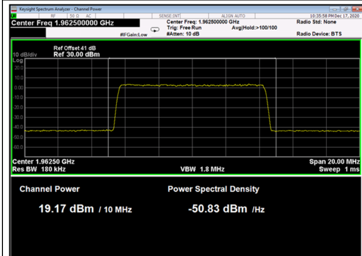
Figure 151: 256QAM 10MHz B.W.; 1962.5MHz, 30kHz
