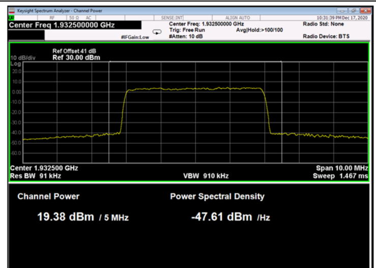
Figure 142: 256QAM 5MHz B.W.; 1932.5MHz, 30kHz
