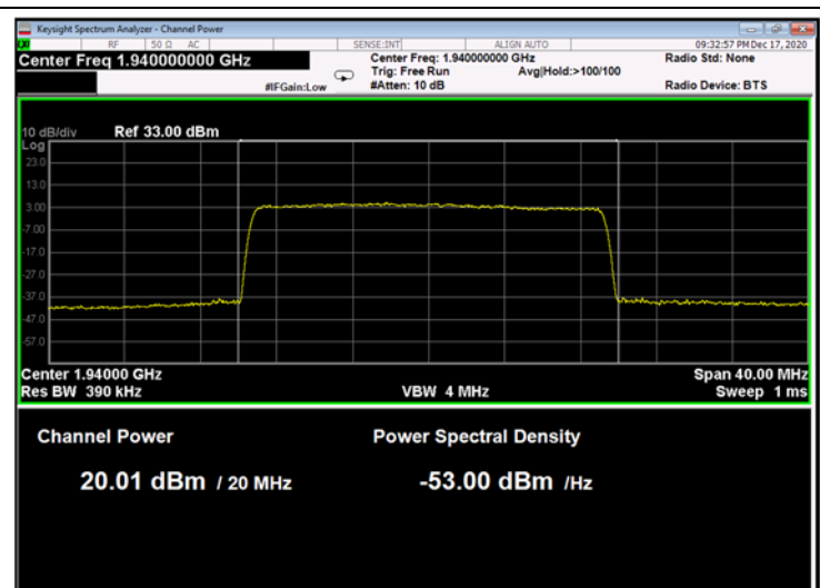
Figure 100: 64QAM 20MHz B.W.; 1940.0MHz, 30kHz
