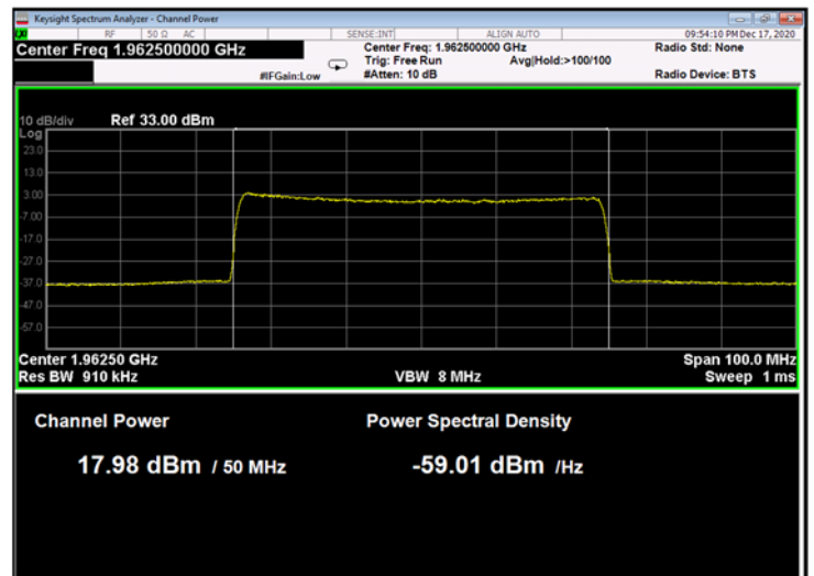
Figure 130: 64QAM 50MHz B.W.; 1962.5MHz, 30kHz
