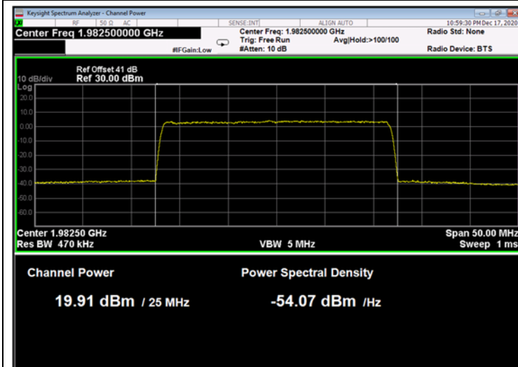
Figure 181: 256QAM 25MHz B.W.; 1982.5MHz, 30kHz
