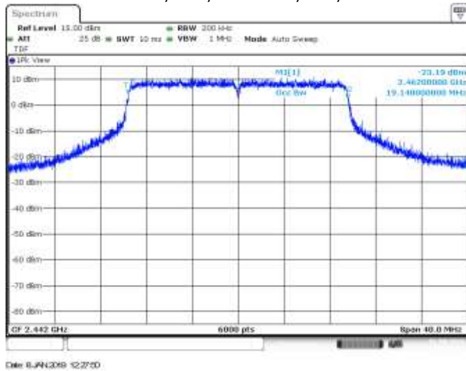
SISO A, CH7, 802.11he20, HE0, 99%
