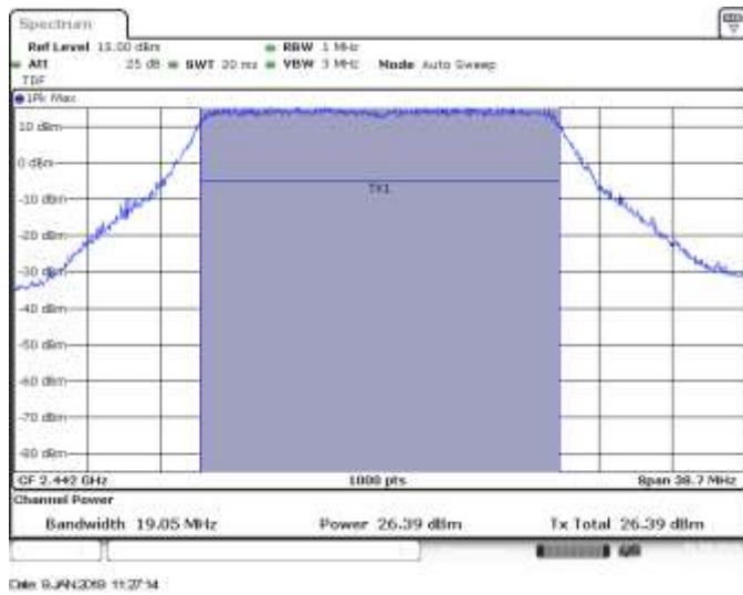
MIMO A, CH7, 802.11he20, HE0
