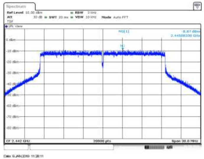
MIMO A, CH7, 802.11he20, HE0
