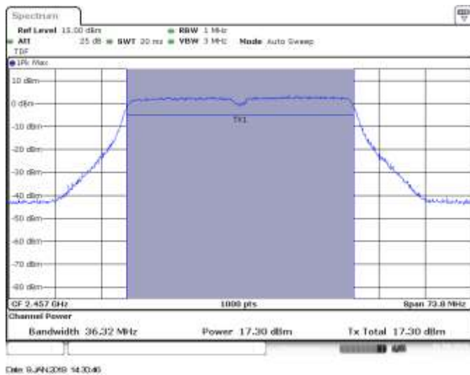
MIMO B, CH10, 802.11n40, HT8
