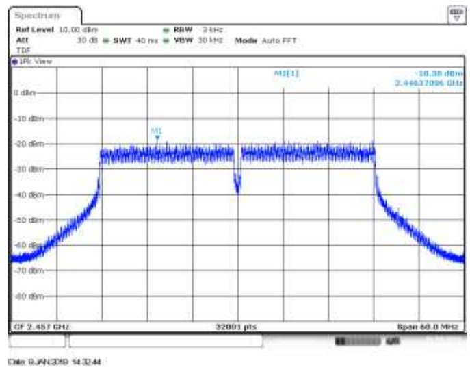
MIMO B, CH10, 802.11n40, HT8
