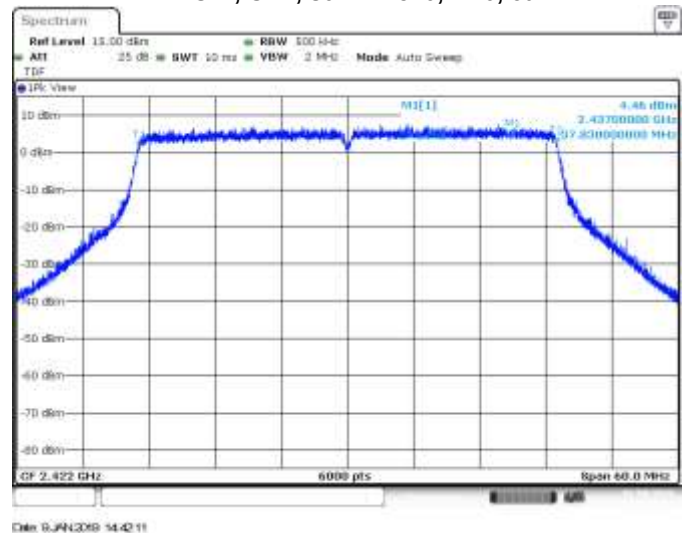
MIMO B, CH3, 802.11he40, HE0, 99%
