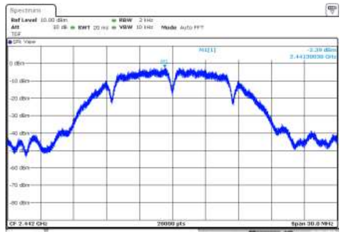
SISO A, CH7, 802.11b, 1Mbps
