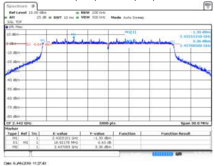
MIMO A, CH7, 802.11he20, HE0, 6dB
