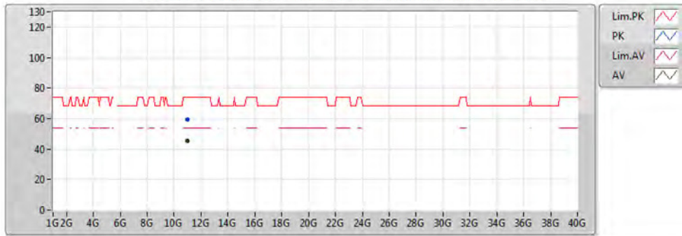
RE TX above 1GHz;Band:5.6G;VHT20;BWch:20MHz;Nss:1,(M0);Nant:4;Ch:5500MHz;TX
