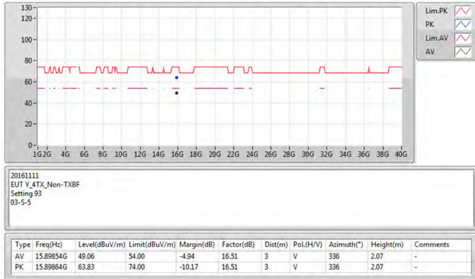
RE TX above 1GHz;Band:5.3G;VHT20;BWch:20MHz;Nss:1.(M0);Nant:4;Ch:5300MHz;TX
