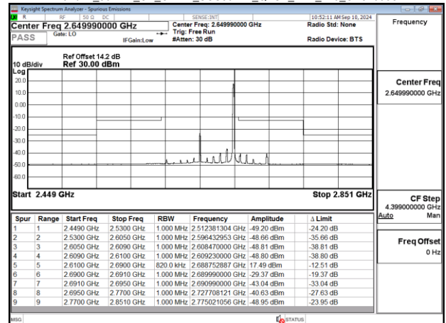
Band41_80MHz_CP_OFDM_SCS30kHz_QPSK_RB1_216_CH529998
