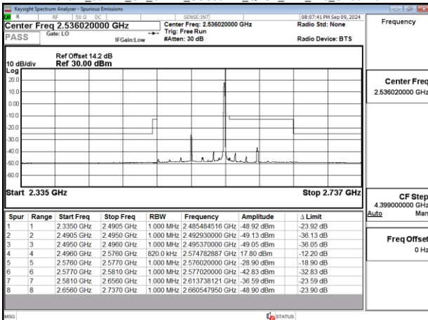
Band41_80MHz_CP_OFDM_SCS30kHz_QPSK_RB1_216_CH507204
