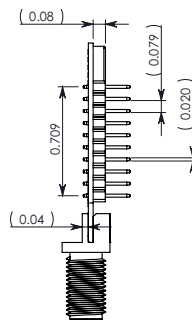
RPSMA
