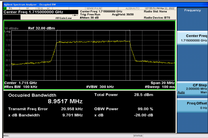
Band4-10MHz-QPSK-20000-50RB#0-8.9517
