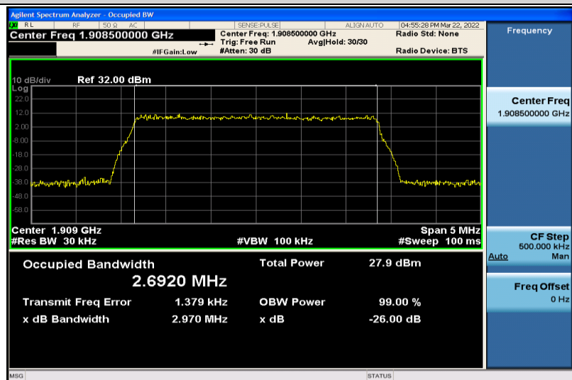
Band2-3MHz-QPSK-19185-15RB#0-2.6920
