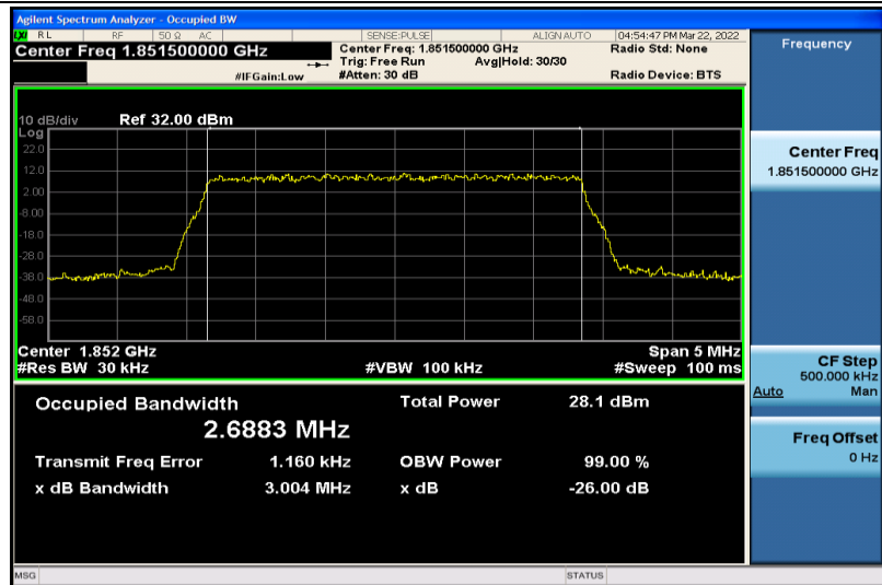
Band2-3MHz-QPSK-18615-15RB#0-2.6883
