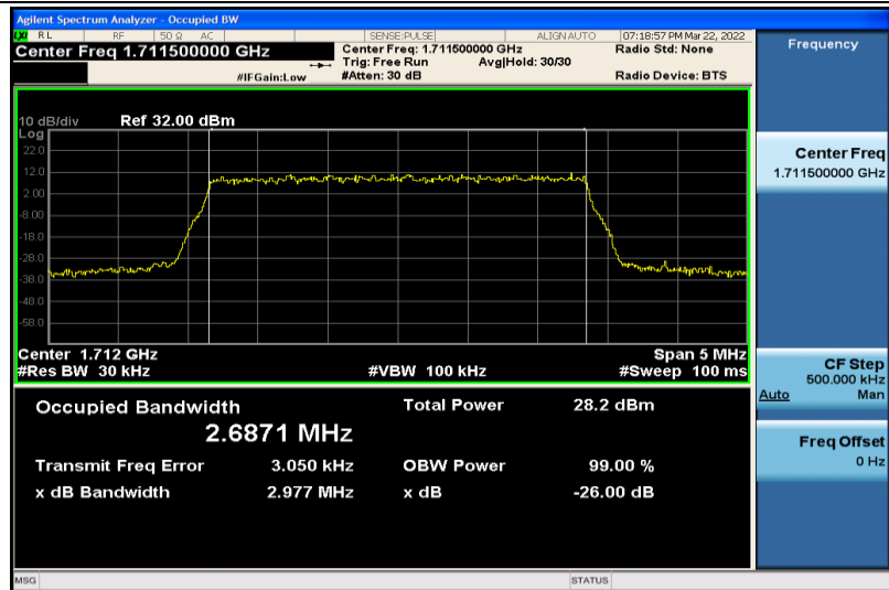
Band4-3MHz-QPSK-19965-15RB#0-2.6871
