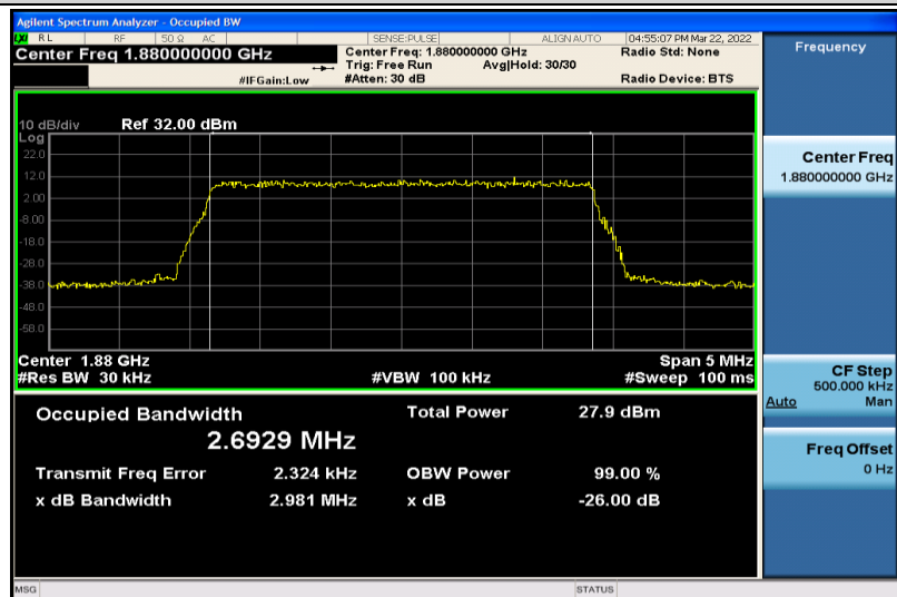
Band2-3MHz-QPSK-18900-15RB#0-2.6929
