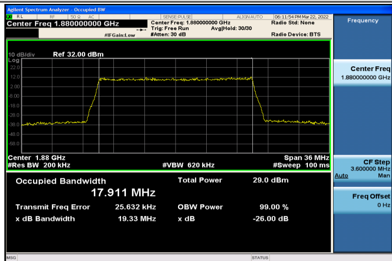
Band2-20MHz-QPSK-18900-100RB#0-17.911
