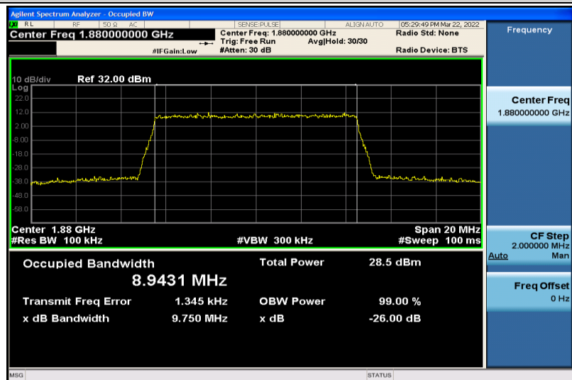
Band2-10MHz-QPSK-18900-50RB#0-8.9431
