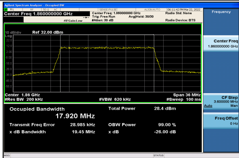
Band2-20MHz-16QAM-18700-100RB#0-17.920
