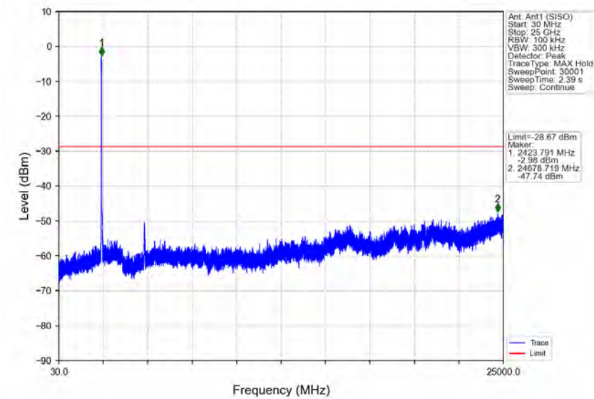
802.11n(HT40)_MCH_2437MHz_Ant1 (SISO)_NTNV
