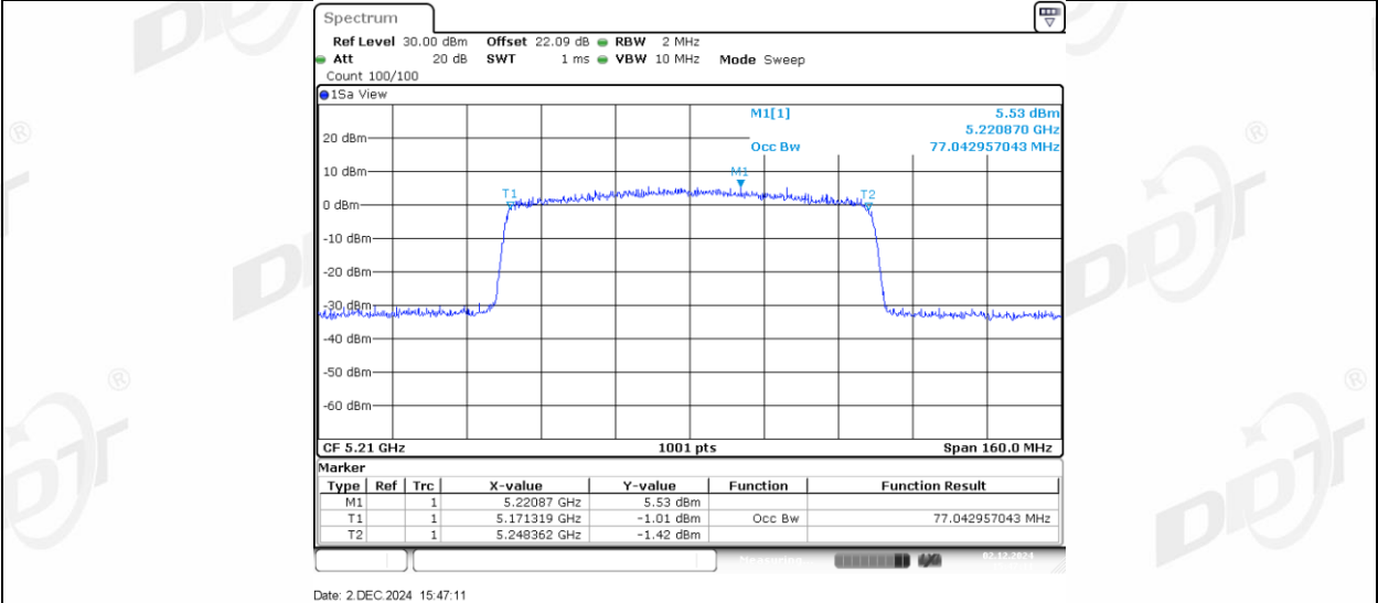
11AX80MIMO_Ant2_5210
