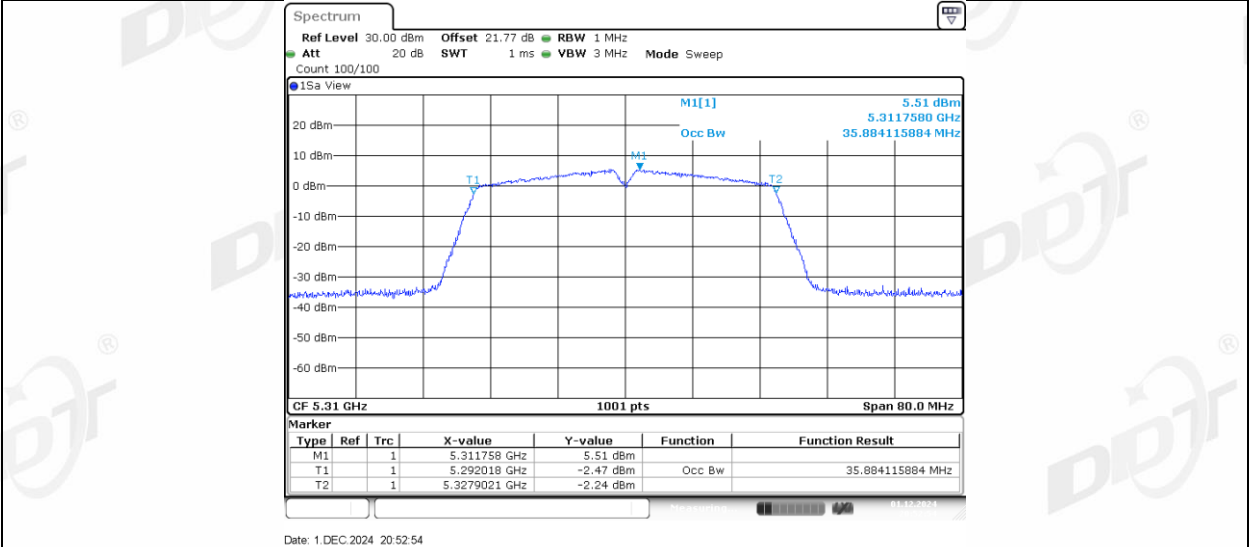
11AC40MIMO_Ant2_5310
