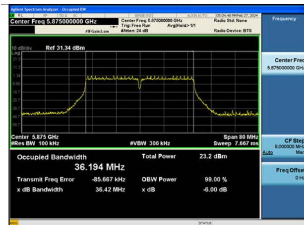
802.11ac(VHT40) (CH.175)
