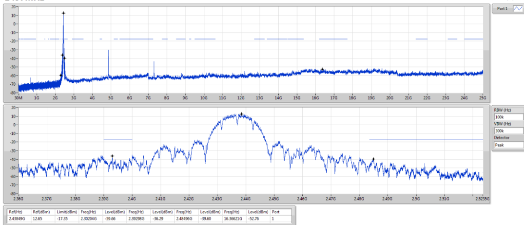
802.11b_Nss1,(1Mbps)_1TX 2437MHz
