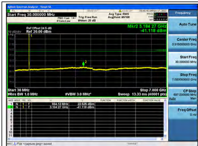
Band71 / 15MHz / High CH / QPSK
