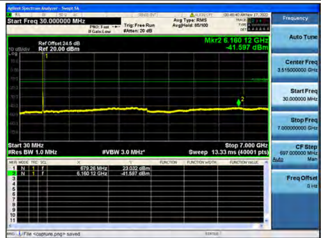
Band71 / 20MHz / High CH / QPSK
