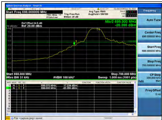
Band12 / 5MHz / Low CH / QPSK / 1 RB
