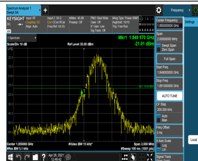
EGPRS1900-512-2
