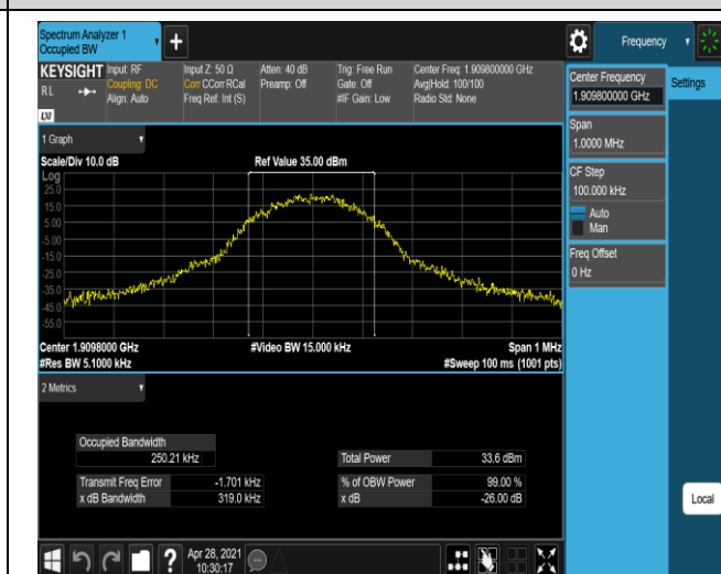
EGPRS1900-810-2-0.3190
