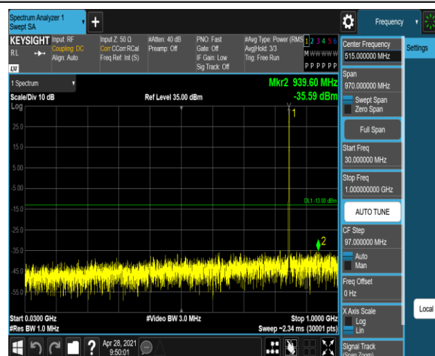
GSM850-190-3-30~1000MHz
