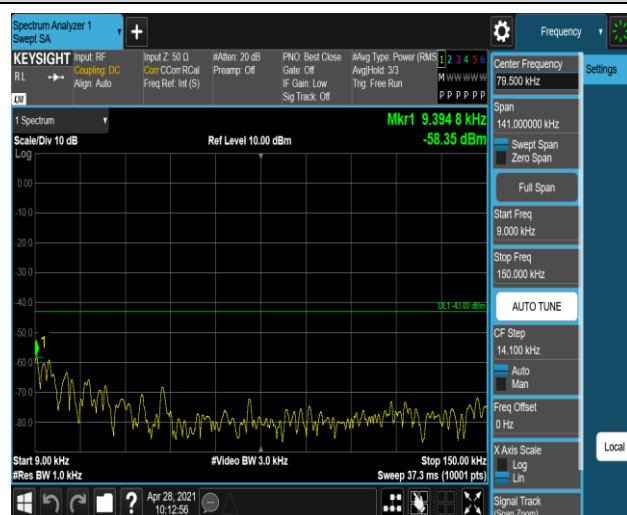
GSM1900-512-0-0.009~0.15MHz
