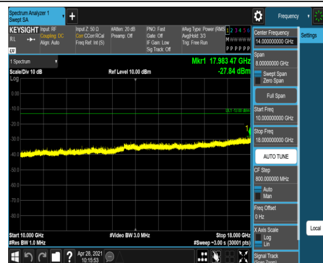
GSM1900-661-0-10000~18000MHz
