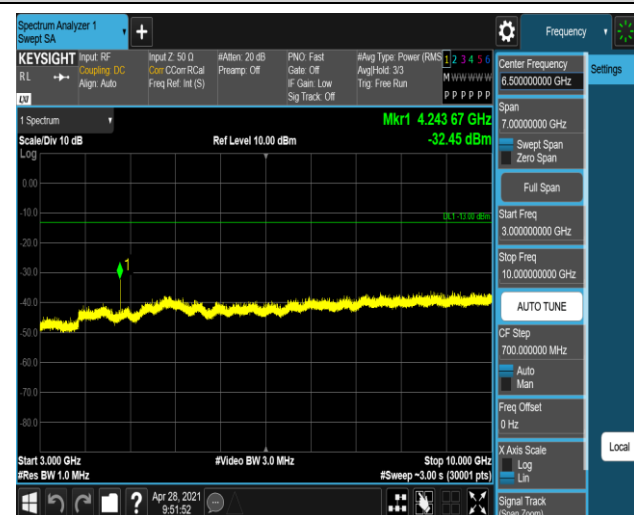
GSM850-251-3-3000~10000MHz
