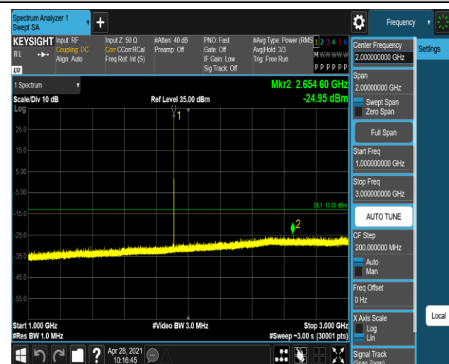
GSM1900-810-0-1000~3000MHz
