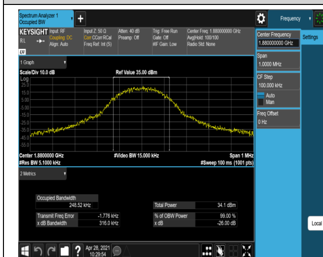
EGPRS1900-661-2-0.3160
