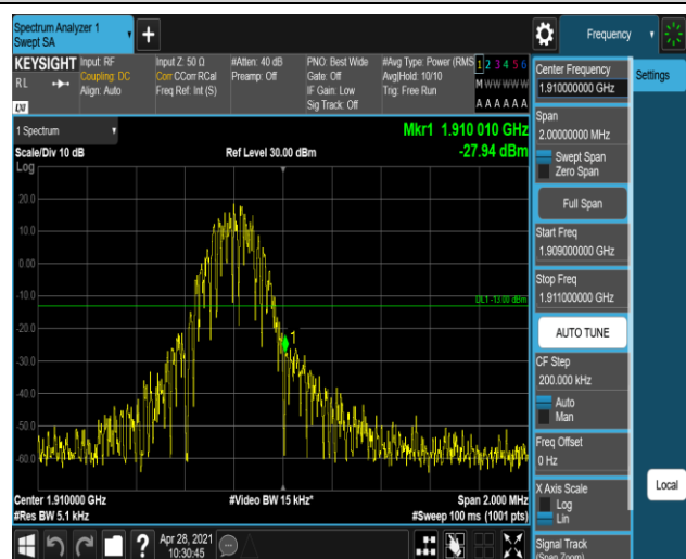
EGPRS1900-810-2
