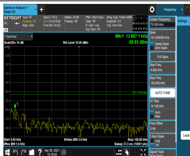
GSM1900-810-0-0.009~0.15MHz
