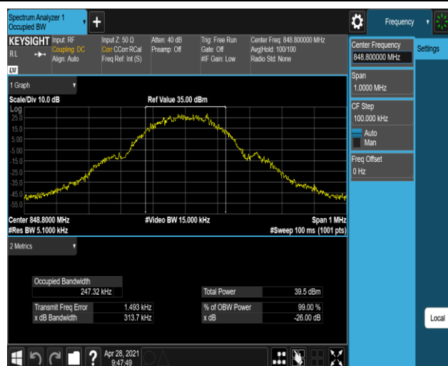
GSM850-251-3-0.3137
