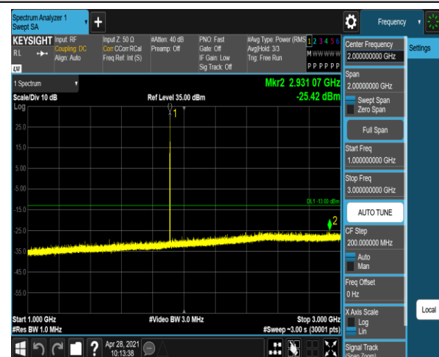
GSM1900-512-0-1000~3000MHz
