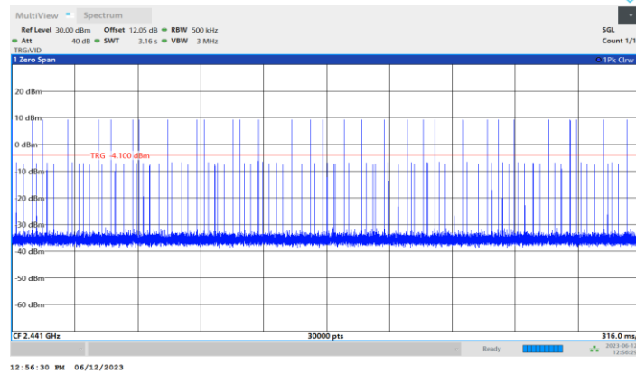
3DH1_Ant1_Hop
