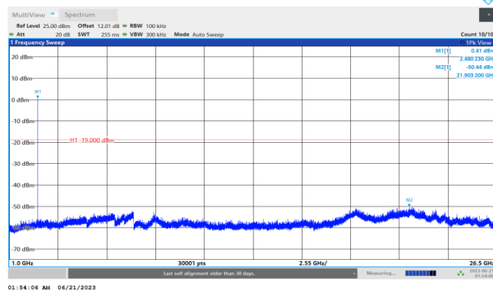
DH5_Ant1_2480_1000~26500
