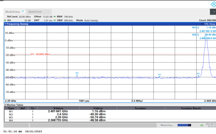
DH5_Ant1_Low_2402
