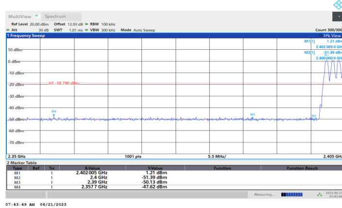
DH5_Ant1_Low_Hop_2402
