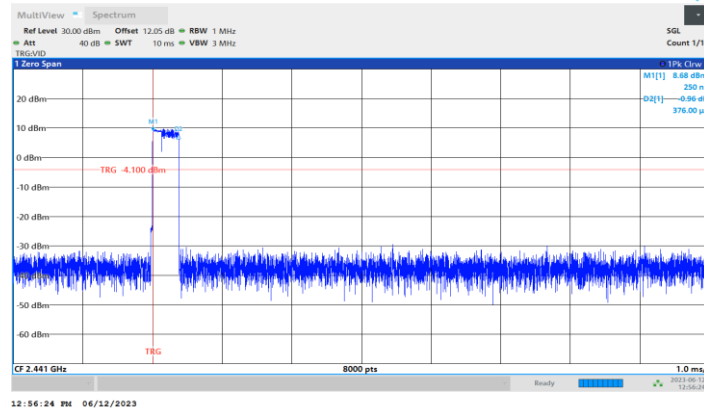
3DH1_Ant1_Hop
