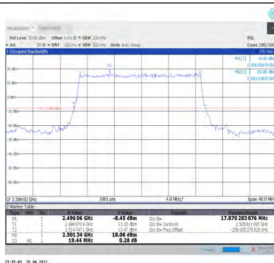
1-N41--30-20-L-2-DFT-PI2BPSK-Outer_Full-50@0-Ant1 -17.87-19.440-≤20-PASS
