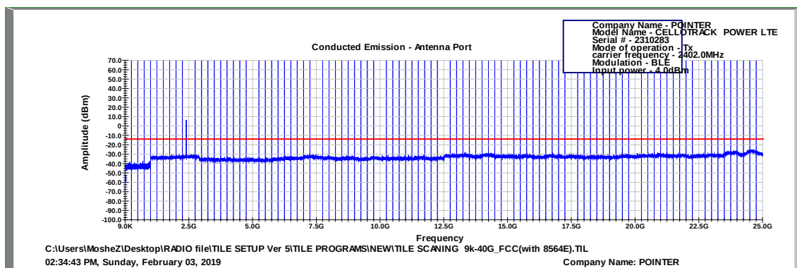
Figure 35 2402.0 MHz, BLE
