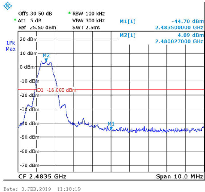
Figure 23 Band Edge High, BLE
