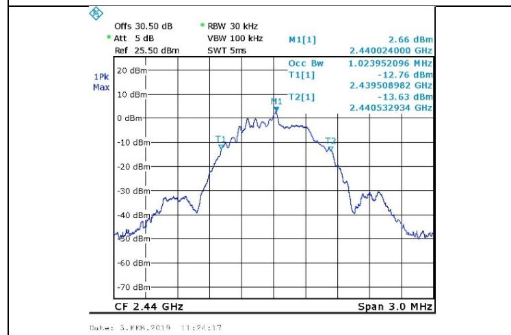
Figure 32. 2440.0 MHz, BLE
