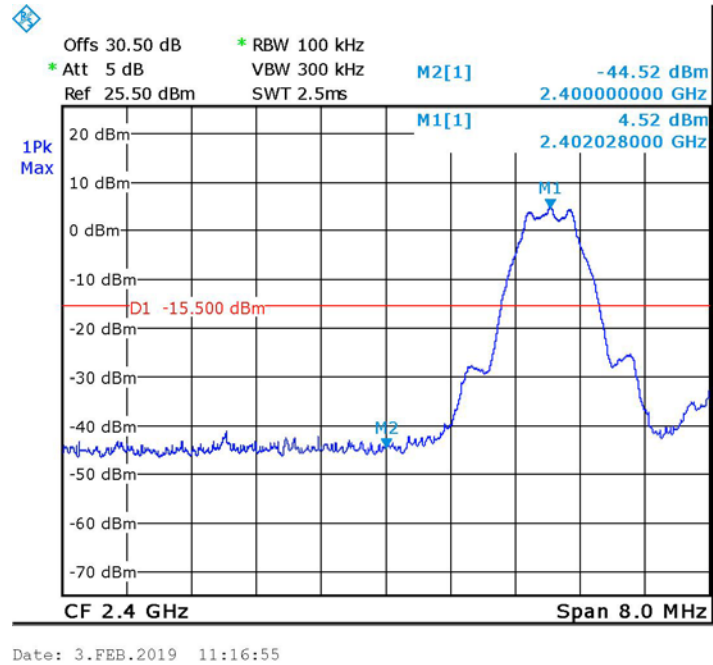
Figure 22 Band Edge Low, BLE
