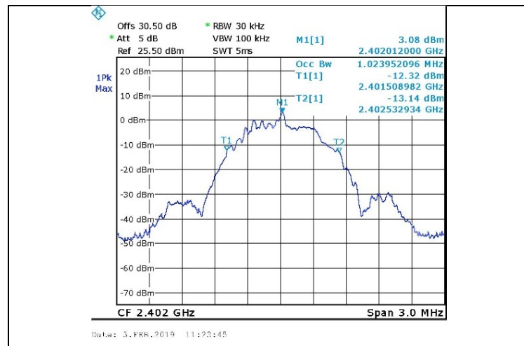
Figure 31. 2402.0 MHz, BLE
