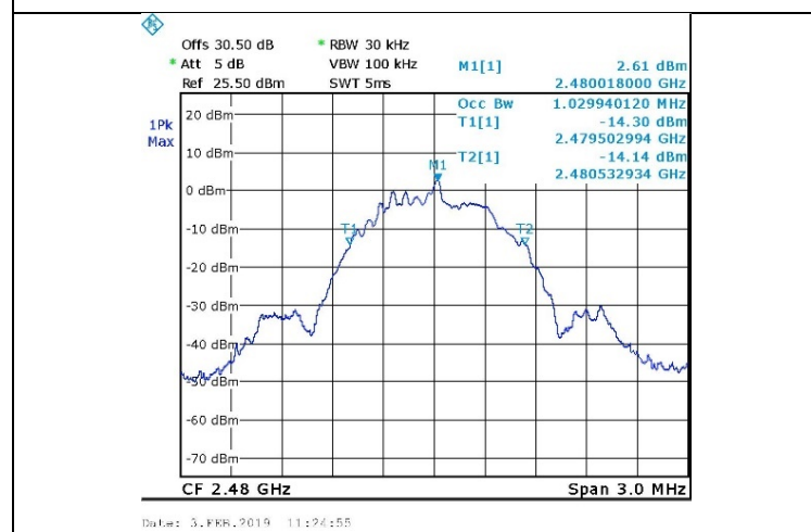
Figure 33. 2480.0 MHz, BLE
