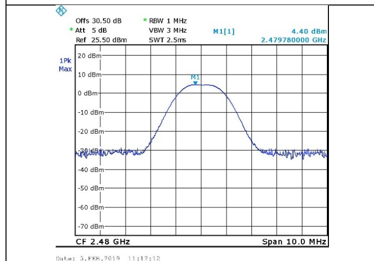
Figure 19. 2480.0 MHz, BLE
