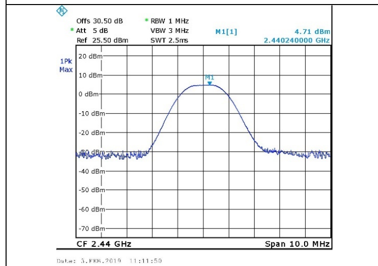
Figure 18. 2440.0 MHz, BLE
