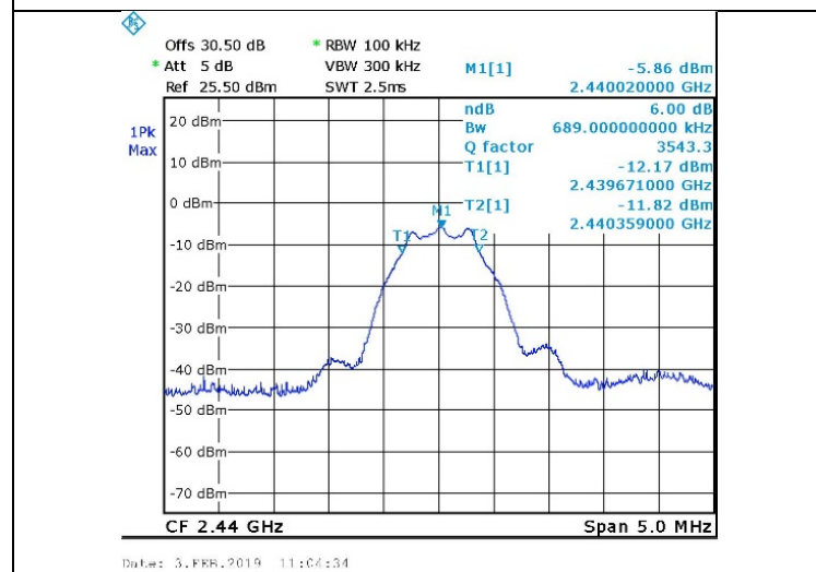
Figure 13. 2440.0 MHz, BLE
