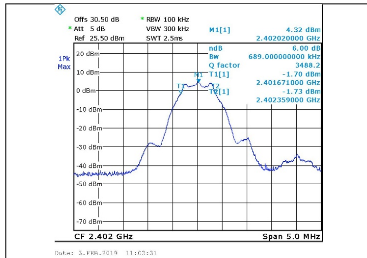
Figure 12. 2402.0 MHz, BLE
