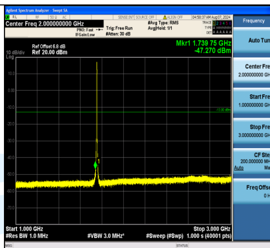
Band4 5MHz QPSK 20375 25RB#0 1000~3000 1000~3000
