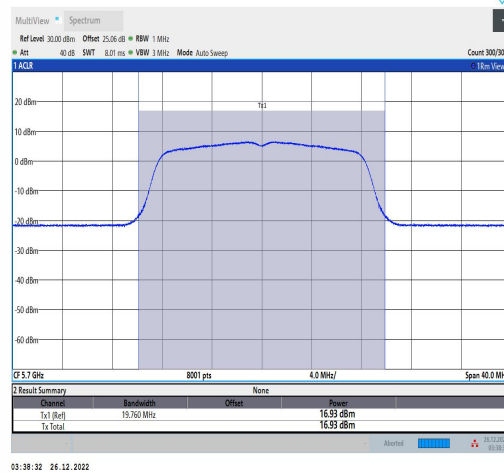
11A-Ant1-5700-TPC L-----16.78-96.55-0.15
