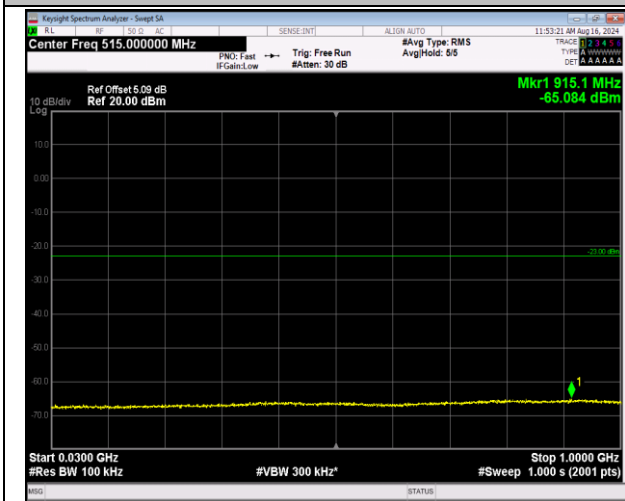
66-66-5MHz-20MHz-16QAM-16QAM-132455-132572-1R B#0-1RB#99-30~1000MHz-PASS
