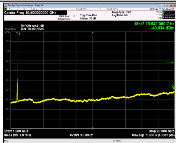
66-66-20MHz-5MHz-QPSK-QPSK-132397-132514-1RB#0- ORB#0-1000~20000MHz-PASS
