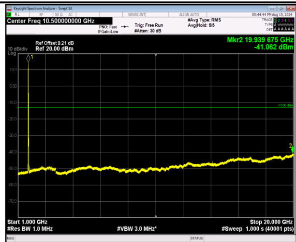
66-66-20MHz-5MHz-QPSK-QPSK-132072-132189-1RB#0- 1RB#24-1000~20000MHz-PASS
