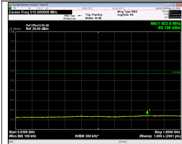
66-66-20MHz-20MHz-QPSK-QPSK-132072-132270-1RB #0-ORB#0-30~1000MHz-PASS
