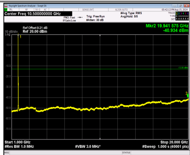
66-66-20MHz-5MHz-QPSK-QPSK-132072-132189-1RB#0- ORB#0-1000~20000MHz-PASS
