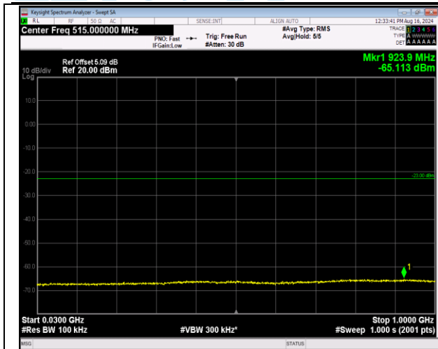
66-66-5MHz-20MHz-64QAM-64QAM-132455-132572-1R B#24-ORB#0-30~1000MHz-PASS
