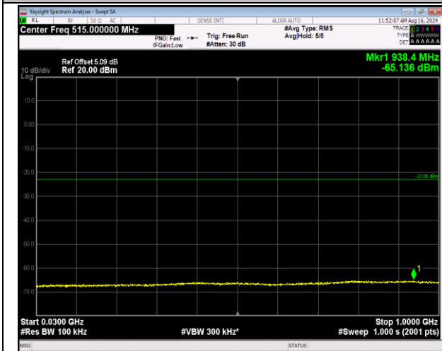
66-66-5MHz-20MHz-16QAM-16QAM-132455-132572-1R B#24-0RB#0-30~1000MHz-PASS
