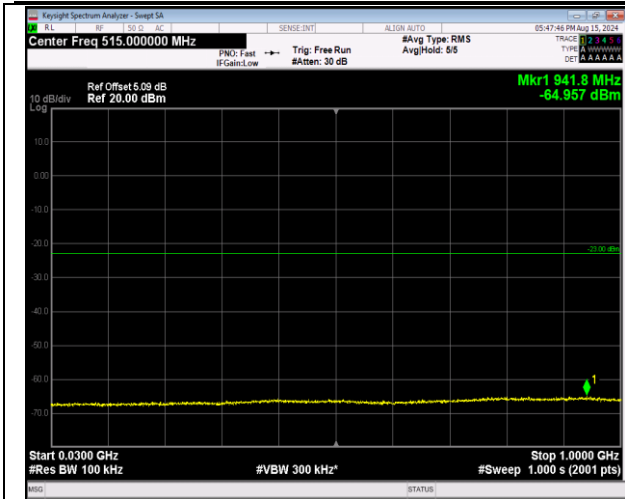
66-66-20MHz-5MHz-16QAM-16QAM-132397-132514-1R B#0-0RB#0-30~1000MHz-PASS
