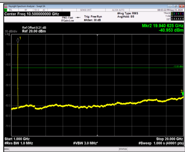
66-66-20MHz-5MHz-64QAM-64QAM-132072-132189-100R B#0-25RB#0-1000~20000MHz-PASS
