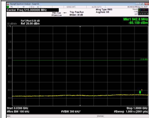
66-66-20MHz-5MHz-16QAM-16QAM-132397-132514-1R B#99-0RB#0-30~1000MHz-PASS
