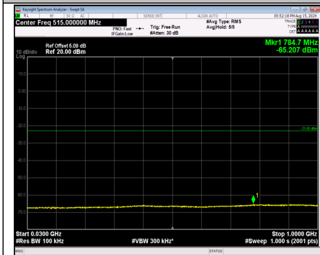
66-66-20MHz-5MHz-QPSK-QPSK-132522-132639-1RB# 0-ORB#0-30~1000MHz-PASS
