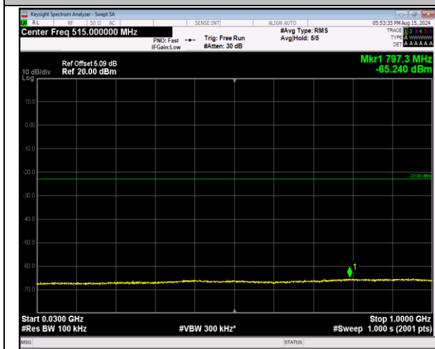
66-66-20MHz-5MHz-QPSK-QPSK-132522-132639-1RB# 99-0RB#0-30~1000MHz-PASS
