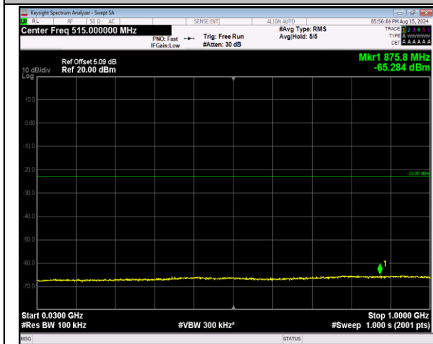
66-66-20MHz-5MHz-QPSK-QPSK-132522-132639-100R B#0-25RB#0-30~1000MHz-PASS
