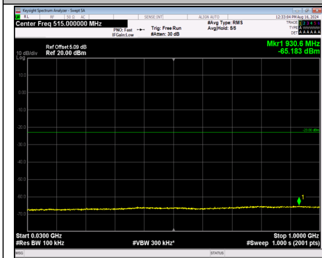
66-66-5MHz-20MHz-64QAM-64QAM-132455-132572-1R B#0-0RB#0-30~1000MHz-PASS
