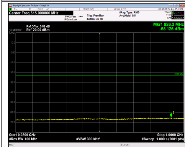
66-66-20MHz-5MHz-QPSK-QPSK-132397-132514-100RB B#0-25RB#0-30-1000MHz-PASS
