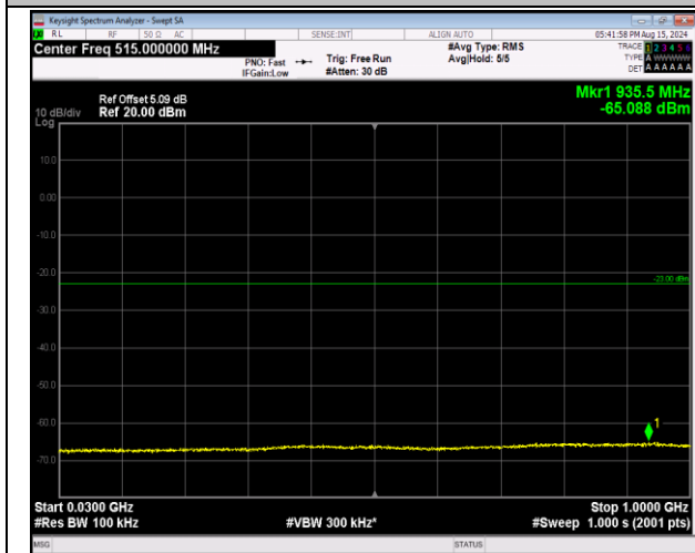
66-66-20MHz-5MHz-QPSK-QPSK-132072-132189-1RB# 0-ORB#0-30~1000MHz-PASS
