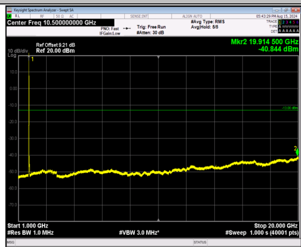
66-66-20MHz-5MHz-QPSK-QPSK-132072-132189-1RB#99 -0RB#0-1000~20000MHz-PASS
