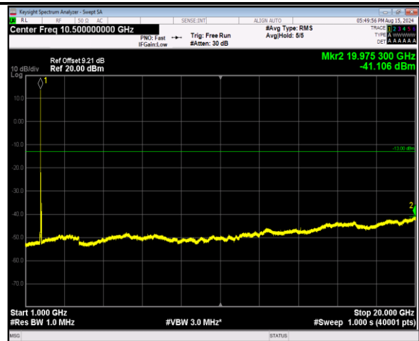
66-66-20MHz-5MHz-QPSK-QPSK-132397-132514-1RB#0- 1RB#24-1000-20000MHz-PASS
