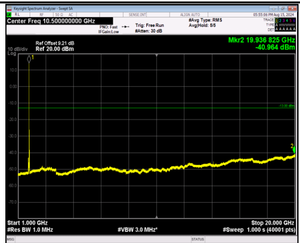
66-66-20MHz-5MHz-QPSK-QPSK-132522-132639-1RB#0- 1RB#24-1000~20000MHz-PASS
