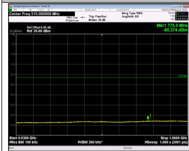
66-66-20MHz-5MHz-QPSK-QPSK-132072-132189-1RB# 99-0RB#0-30~1000MHz-PASS
