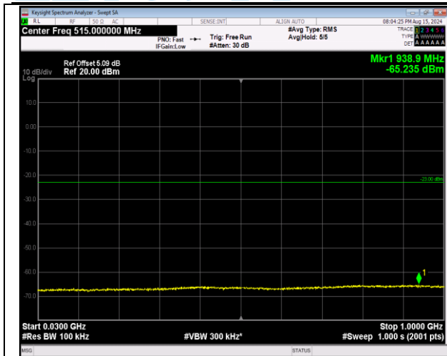
66-66-20MHz-5MHz-64QAM-64QAM-132397-132514-1R B#99-ORB#0-30~1000MHz-PASS
