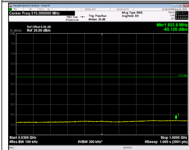
66-66-5MHz-20MHz-64QAM-64QAM-132455-132572-1R B#0-1RB#99-30~1000MHz-PASS
