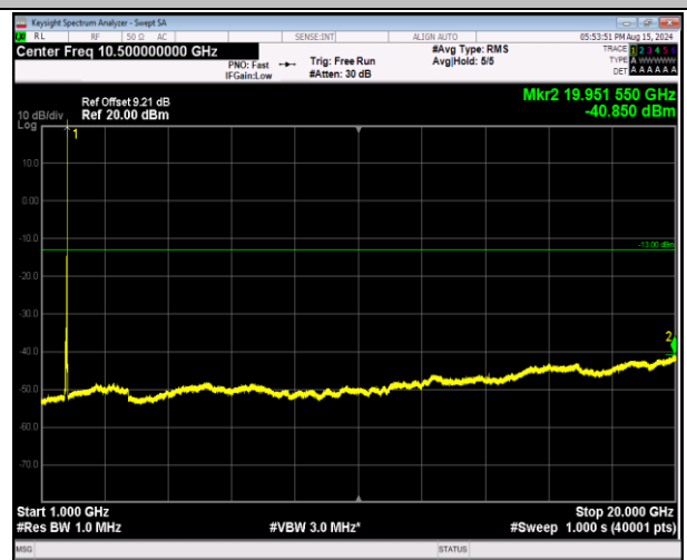
66-66-20MHz-5MHz-QPSK-QPSK-132522-132639-1RB#99 -0RB#0-1000~20000MHz-PASS
