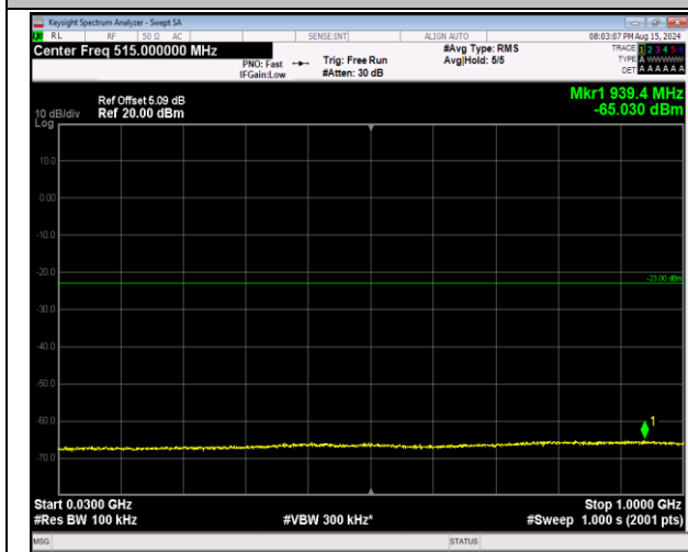
66-66-20MHz-5MHz-64QAM-64QAM-132072-132189-10 ORB#0-25RB#0-30~1000MHz-PASS
