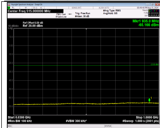
66-66-20MHz-5MHz-QPSK-QPSK-132397-132514-1RB# 0-1RB#24-30-1000MHz-PASS
