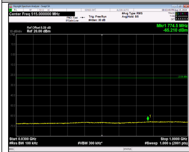
66-66-20MHz-5MHz-64QAM-64QAM-132397-132514-1R B#0-ORB#0-30~1000MHz-PASS
