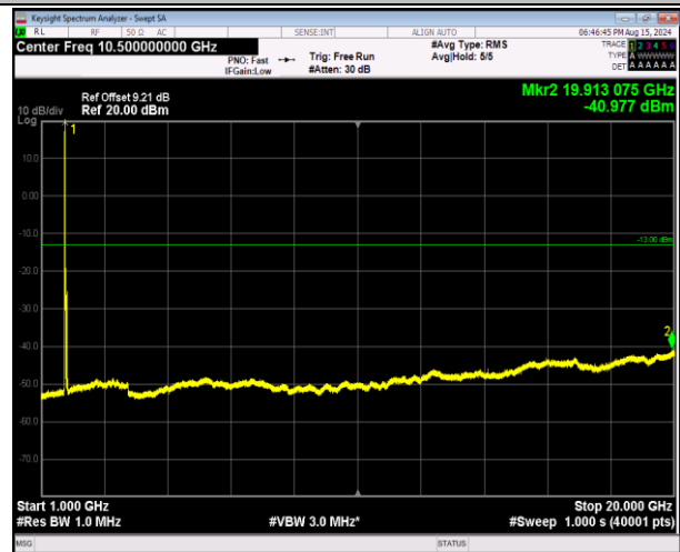
66-66-20MHz-20MHz-QPSK-QPSK-132072-132270-1RB#0 -ORB#0-1000~20000MHz-PASS
