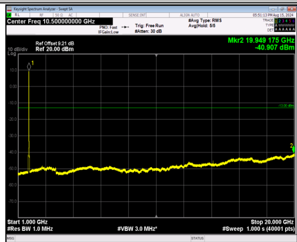
66-66-20MHz-5MHz-QPSK-QPSK-132397-132514-100RB# 0-25RB#0-1000-20000MHz-PASS
