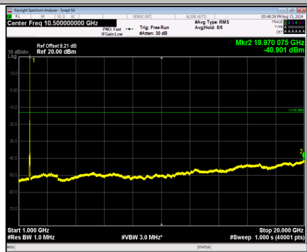
66-66-20MHz-5MHz-QPSK-QPSK-132397-132514-1RB#99 -0RB#0-1000-20000MHz-PASS
