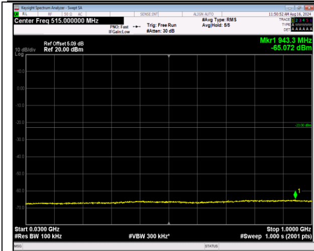
66-66-5MHz-20MHz-16QAM-16QAM-132455-132572-1R B#0-0RB#0-30~1000MHz-PASS
