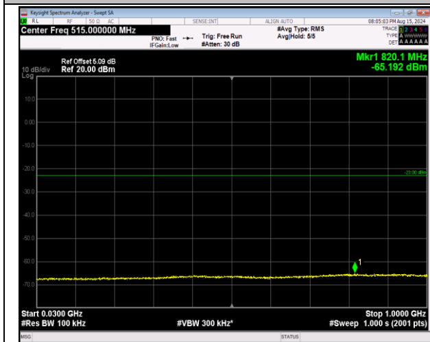
66-66-20MHz-5MHz-64QAM-64QAM-132397-132514-1R B#0-1RB#24-30~1000MHz-PASS
