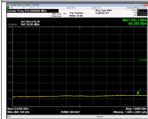
66-66-20MHz-5MHz-QPSK-QPSK-132397-132514-1RB# 99-0RB#0-30-1000MHz-PASS
