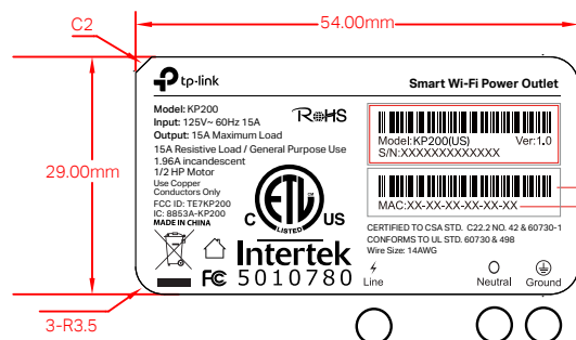
尺寸图 (54.00*29.00mm)
