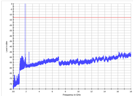
GSM 1900 CH-Middle 30MHz~18GHz
