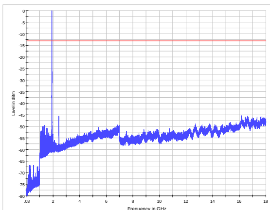
GSM 1900 CH-High 30MHz~18GHz
