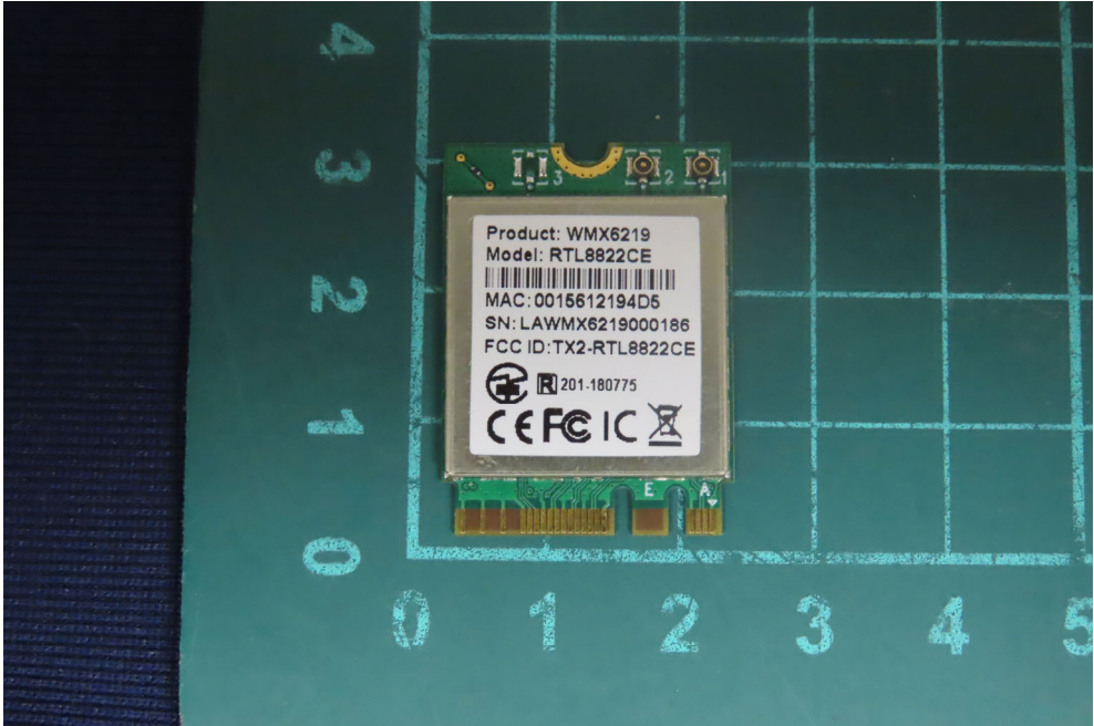
(20) EUT Photo
