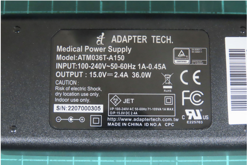
(33) EUT Photo
