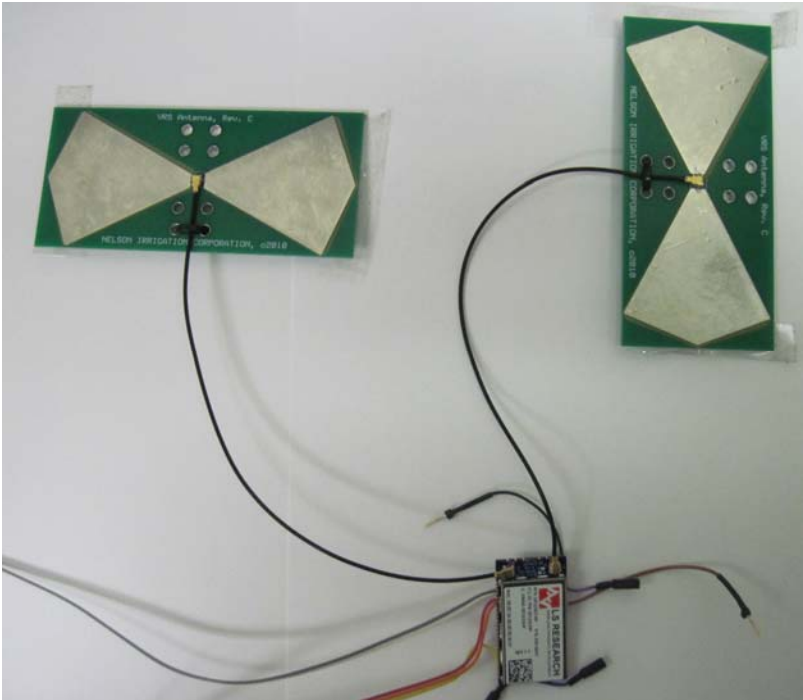
Nelson Bowtie Antenna
