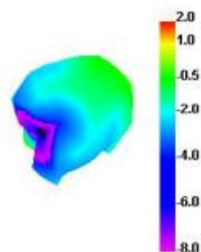
2500.000MHz
