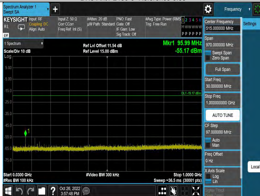
DH5-Ant1-2480-30~1000-0.83
