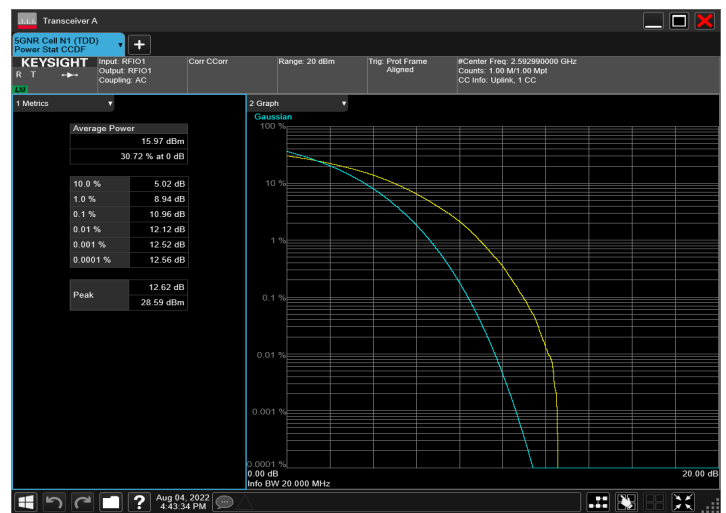
n41_20MHz_30kHz_2592.99MHz_CP-OFDM QPSK_RB51@0
