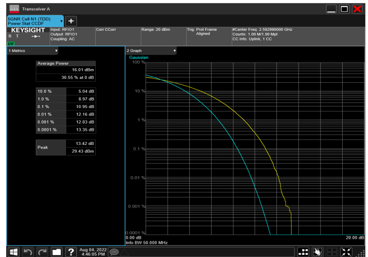
n41_50MHz_30kHz_2592.99MHz_CP-OFDM QPSK_RB133@0
