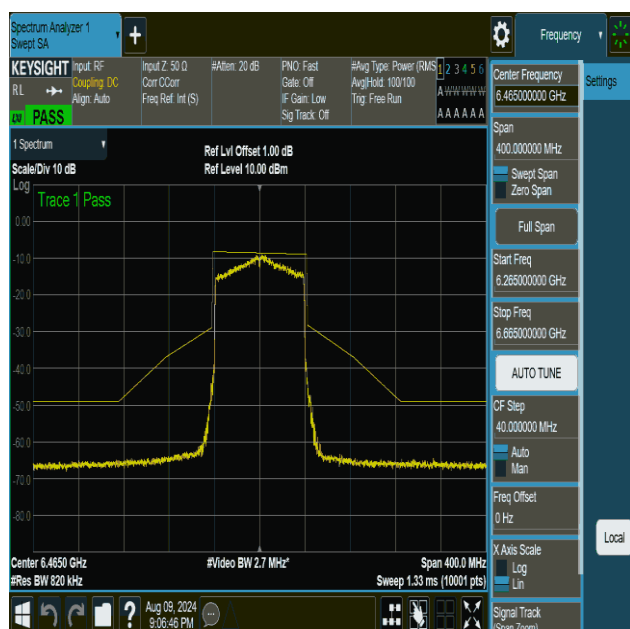
NTVN-11be80MIMO-Ant1-6465-PASS
