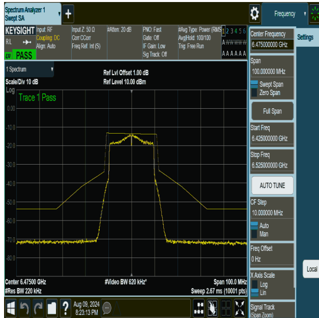
NTVN-11be20MIMO-Ant1-6475-PASS
