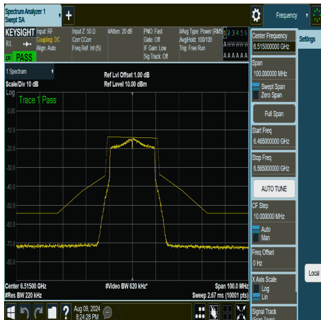
NTVN-11be20MIMO-Ant1-6515-PASS
