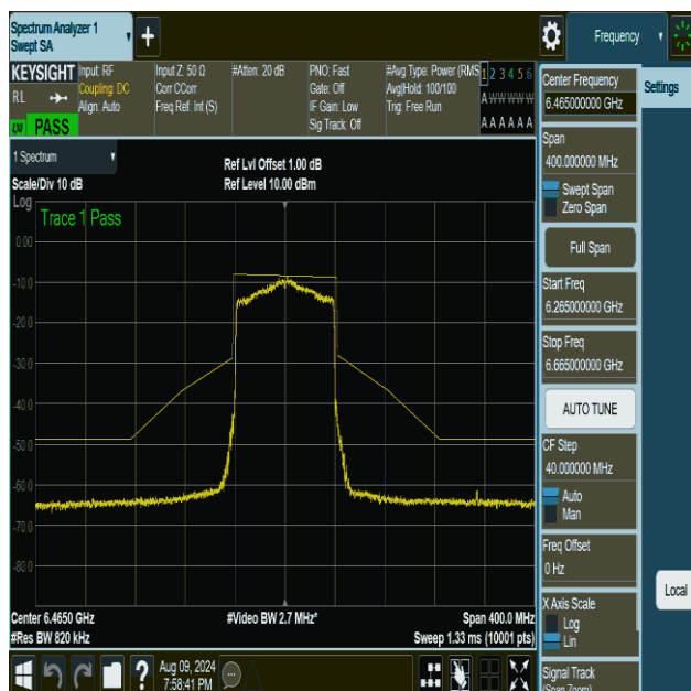
NTVN-11ax80MIMO-Ant1-6465-PASS
