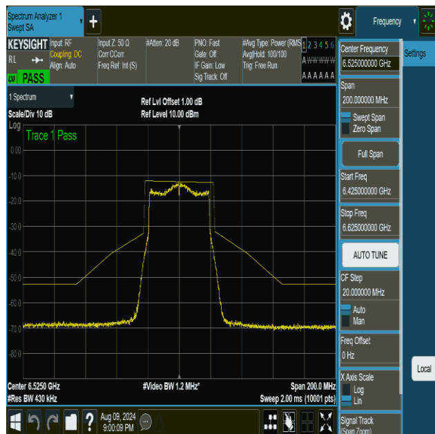
NTVN-11be40MIMO-Ant1-6525-PASS
