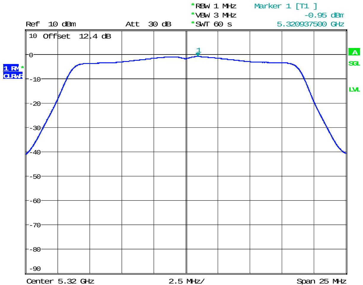
Plot 3. 14 802.11n 20MHz, 5320MHz
