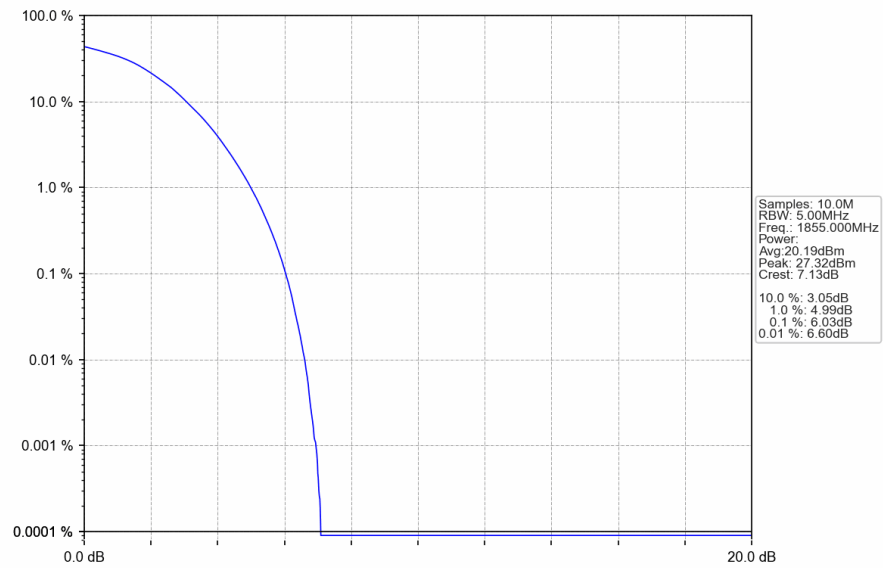
Band2_10MHz_16QAM_LCH_1855MHz_RB_50_0_NTNV
