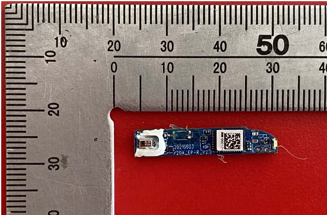
IC Details 2
