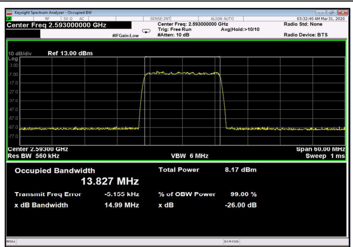
Figure 268: 256QAM 15MHz B.W.; 2593.0MHz, 30kHz Input
