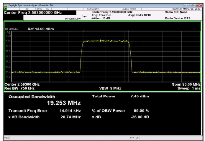
Figure 276: 256QAM 20MHz B.W.; 2593.0MHz, 15kHz Input
