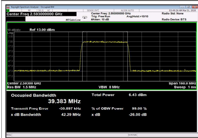
Figure 285: 256QAM 40MHz B.W.; 2593.0MHz, 15kHz Input
