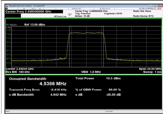
Figure 249: 256QAM 5MHz B.W.; 2498.5MHz, 15kHz Input
