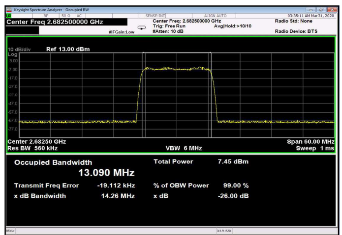
Figure 272: 256QAM 15MHz B.W.; 2682.5MHz, 60kHz Input
