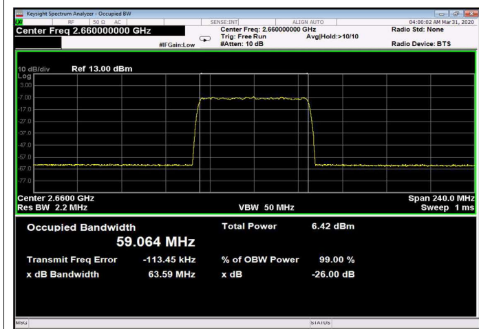
Figure 295: 256QAM 60MHz B.W.; 2660.0MHz, 30kHz Input
