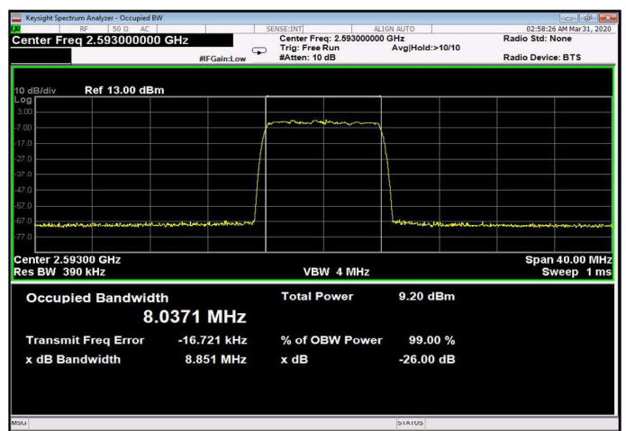
Figure 260: 256QAM 10MHz B.W.; 2593.0MHz, 60kHz Input
