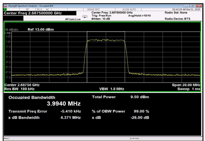
Figure 254: 256QAM 5MHz B.W.; 2687.5MHz, 30kHz Input
