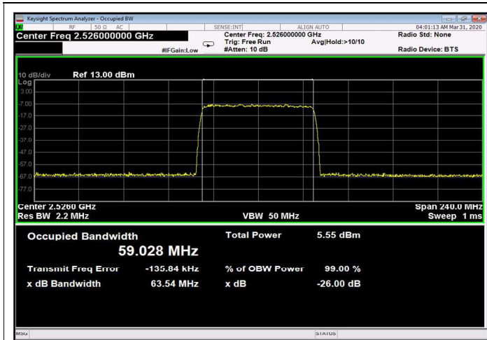
Figure 291: 256QAM 60MHz B.W.; 2526.0MHz, 30kHz Input
