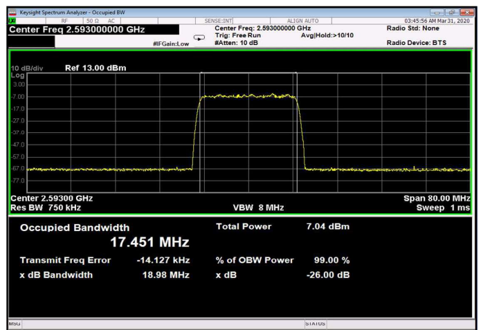
Figure 278: 256QAM 20MHz B.W.; 2593.0MHz, 60kHz Input
