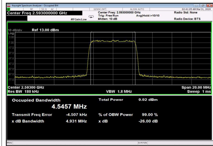
Figure 251: 256QAM 5MHz B.W.; 2593.0MHz, 15kHz Input
