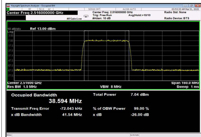
Figure 283: 256QAM 40MHz B.W.; 2516.0MHz, 30kHz Input
