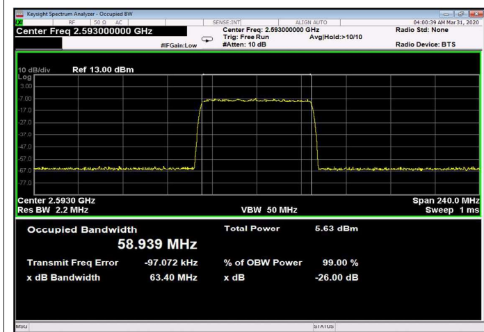
Figure 293: 256QAM 60MHz B.W.; 2593.0MHz, 30kHz Input
