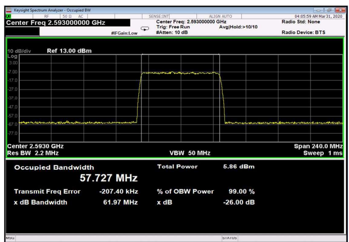
Figure 294: 256QAM 60MHz B.W.; 2593.0MHz, 60kHz Input
