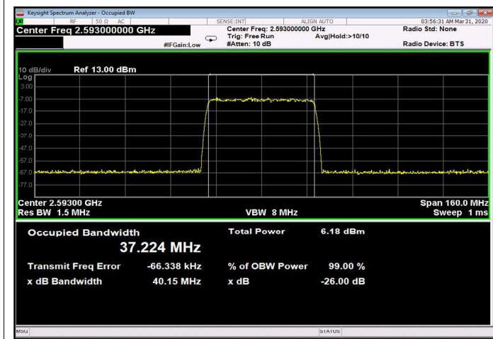
Figure 287: 256QAM 40MHz B.W.; 2593.0MHz, 60kHz Input
