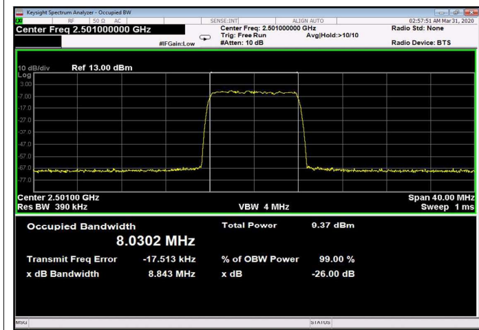
Figure 257: 256QAM 10MHz B.W.; 2501.0MHz, 60kHz Input
