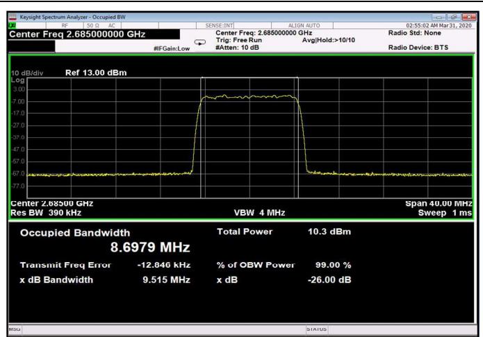
Figure 262: 256QAM 10MHz B.W.; 2685.0MHz, 30kHz Input
