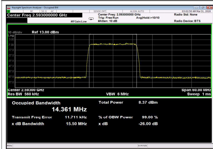
Figure 267: 256QAM 15MHz B.W.; 2593.0MHz, 15kHz Input
