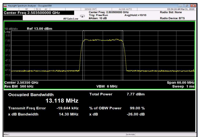
Figure 266: 256QAM 15MHz B.W.; 2503.5MHz, 60kHz Input
