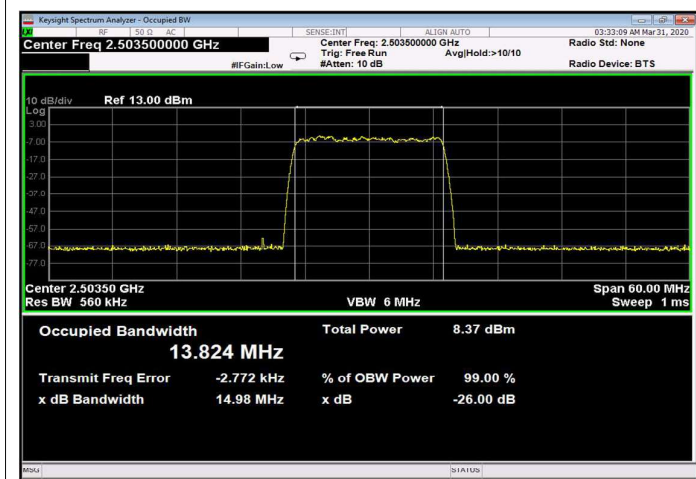
Figure 265: 256QAM 15MHz B.W.; 2503.5MHz, 30kHz Input
