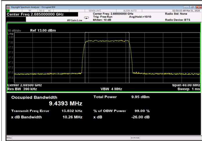
Figure 261: 256QAM 10MHz B.W.; 2685.0MHz, 15kHz Input
