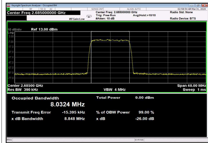
Figure 263: 256QAM 10MHz B.W.; 2685.0MHz, 60kHz Input
