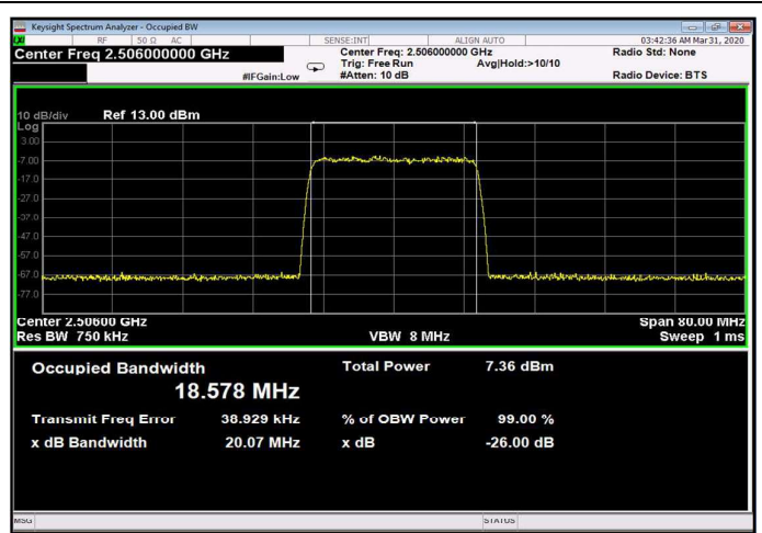
Figure 274: 256QAM 20MHz B.W.; 2506.0MHz, 30kHz Input
