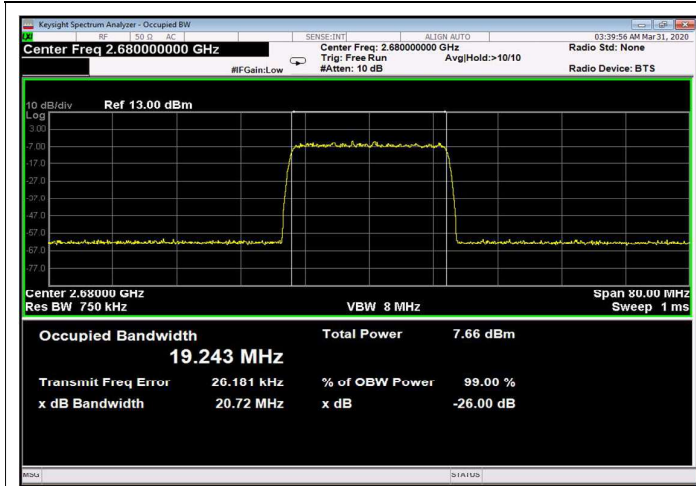
Figure 279: 256QAM 20MHz B.W.; 2680.0MHz, 15kHz Input
