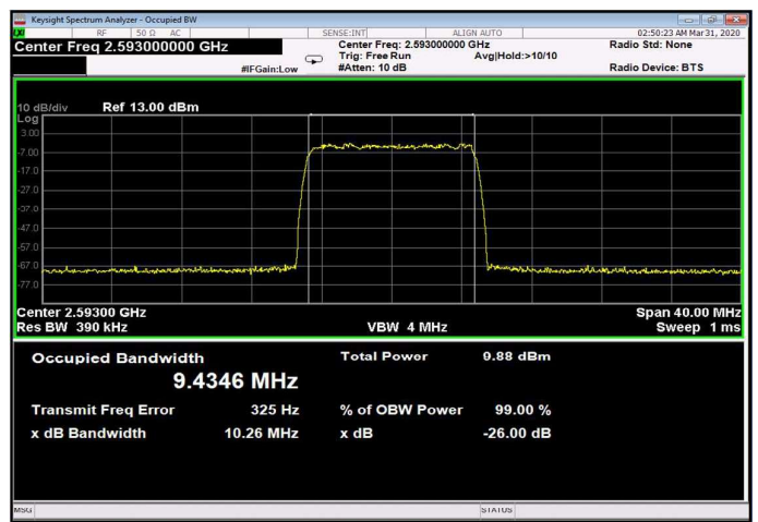
Figure 258: 256QAM 10MHz B.W.; 2593.0MHz, 15kHz Input
