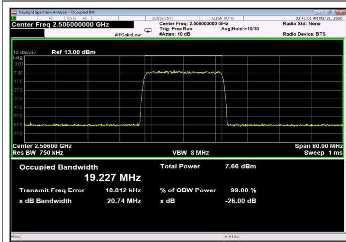
Figure 273: 256QAM 20MHz B.W.; 2506.0MHz, 15kHz Input
