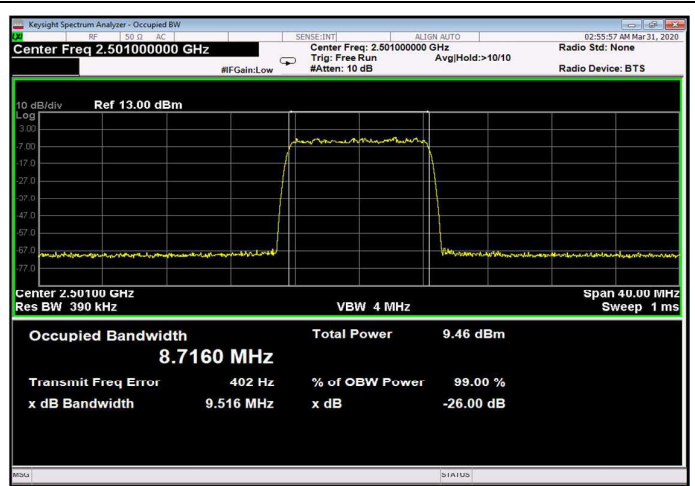
Figure 256: 256QAM 10MHz B.W.; 2501.0MHz, 30kHz Input
