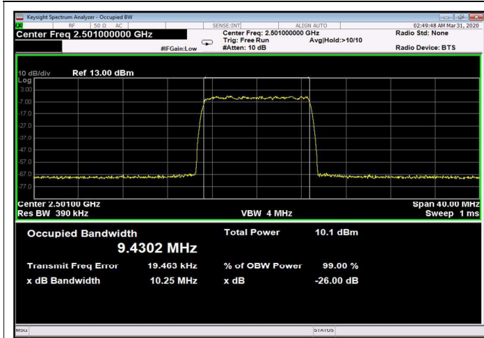
Figure 255: 256QAM 10MHz B.W.; 2501.0MHz, 15kHz Input
