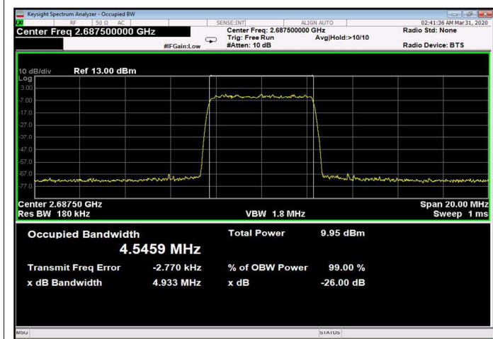
Figure 253: 256QAM 5MHz B.W.; 2687.5MHz, 15kHz Input
