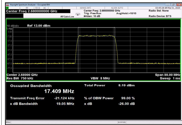
Figure 281: 256QAM 20MHz B.W.; 2680.0MHz, 60kHz Input
