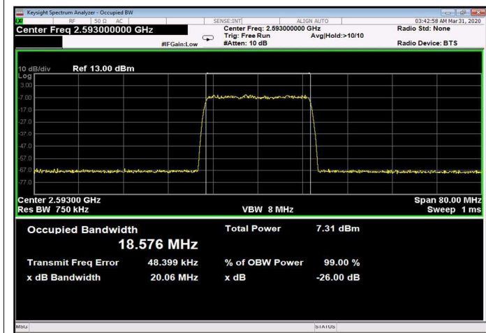
Figure 277: 256QAM 20MHz B.W.; 2593.0MHz, 30kHz Input
