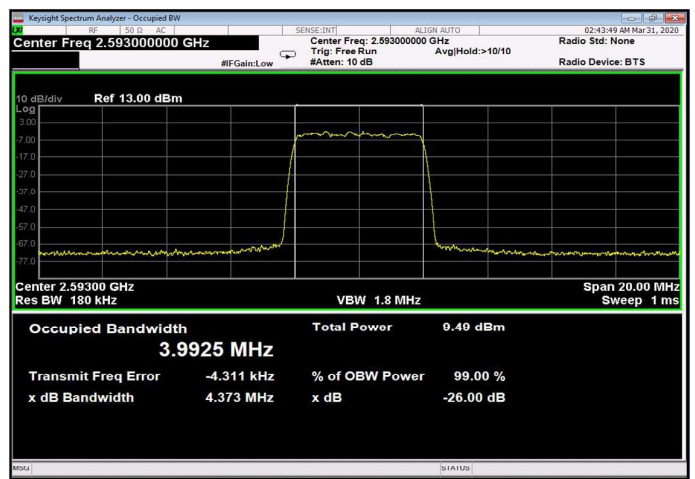
Figure 252: 256QAM 5MHz B.W.; 2593.0MHz, 30kHz Input
