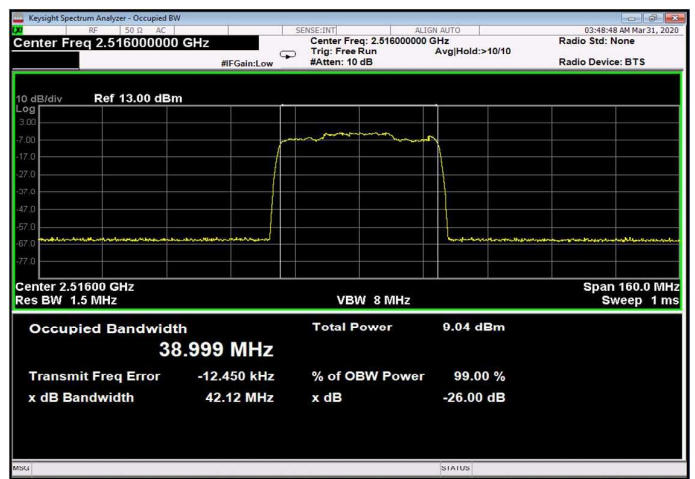
Figure 282: 256QAM 40MHz B.W.; 2516.0MHz, 15kHz Input
