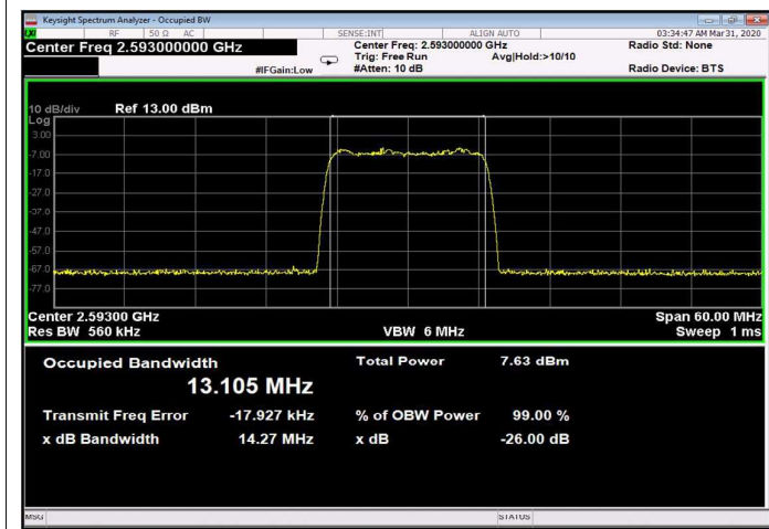
Figure 269: 256QAM 15MHz B.W.; 2593.0MHz, 60kHz Input
