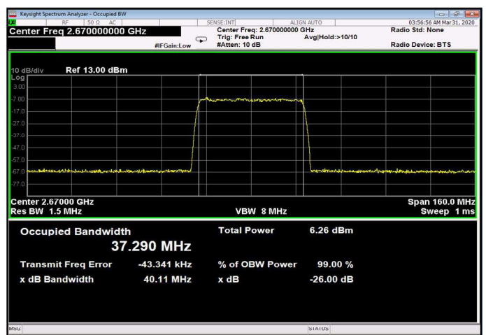
Figure 290: 256QAM 40MHz B.W.; 2670.0MHz, 60kHz Input
