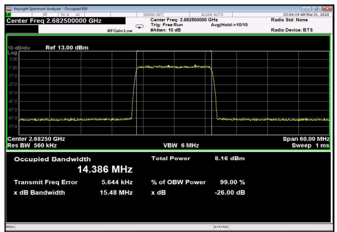
Figure 270: 256QAM 15MHz B.W.; 2682.5MHz, 15kHz Input
