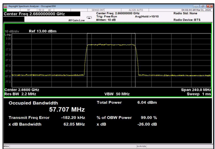
Figure 296: 256QAM 60MHz B.W.; 2660.0MHz, 60kHz Input
