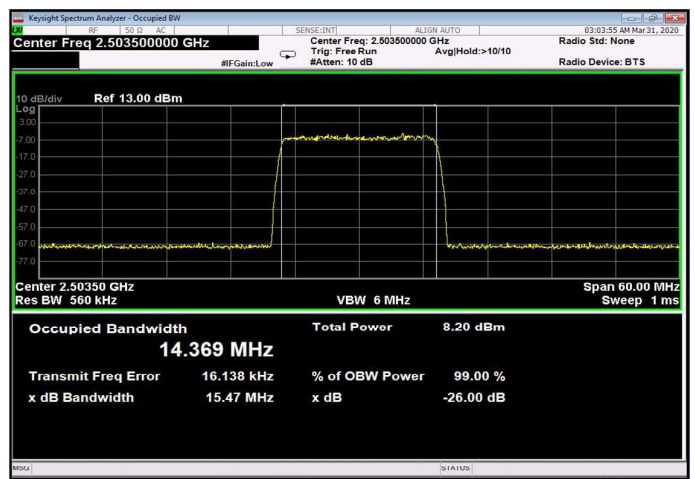
Figure 264: 256QAM 15MHz B.W.; 2503.5MHz, 15kHz Input
