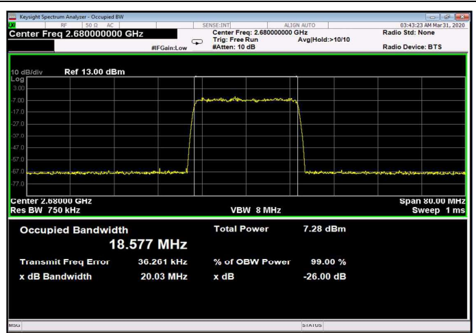
Figure 280: 256QAM 20MHz B.W.; 2680.0MHz, 30kHz Input
