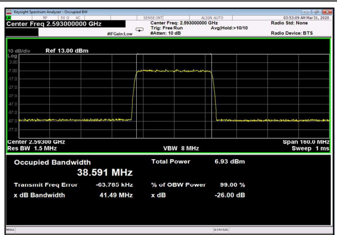
Figure 286: 256QAM 40MHz B.W.; 2593.0MHz, 30kHz Input
