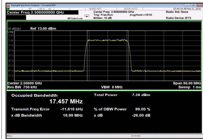
Figure 275: 256QAM 20MHz B.W.; 2506.0MHz, 60kHz Input
