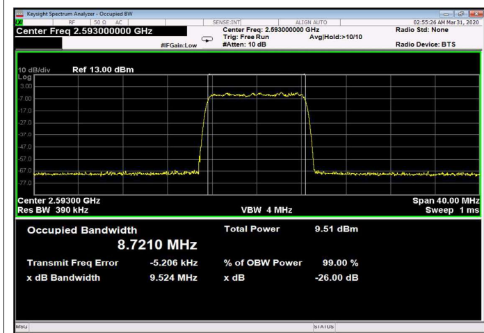
Figure 259: 256QAM 10MHz B.W.; 2593.0MHz, 30kHz Input
