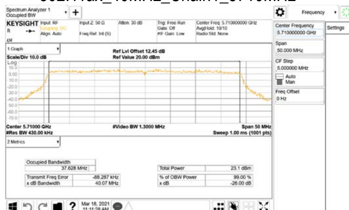
802.11ax_40MHz_Chain1_5710MHz
