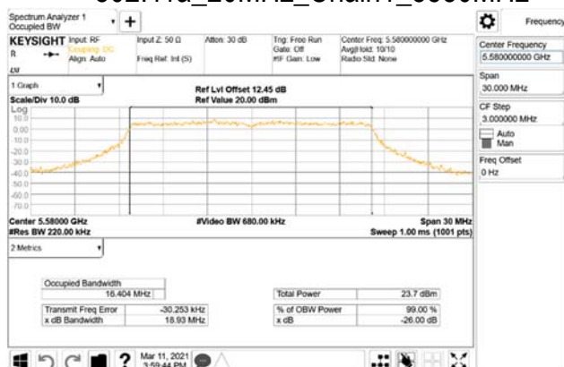
802.11a_20MHz_Chain1_5580MHz
