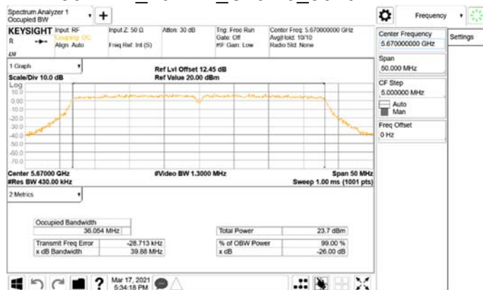
802.11n_40MHz_Chain0_5670MHz
