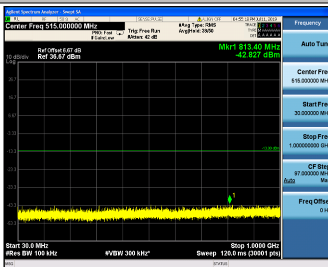
EGPRS1900_661
