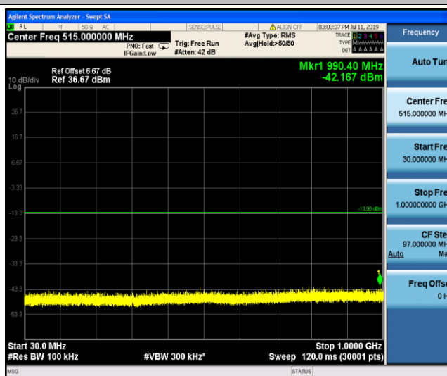
GSM1900_661
