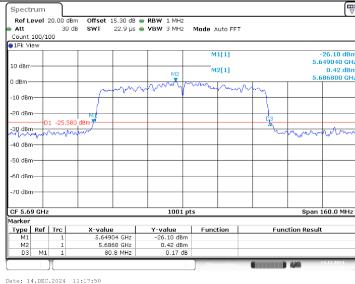
11AC80MIMO_Ant2_5690
