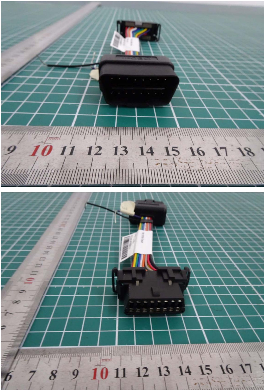
a: Auxiliary cable
