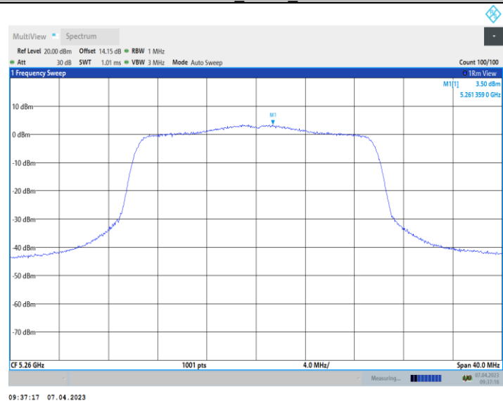
11AX20_Ant10_5280
