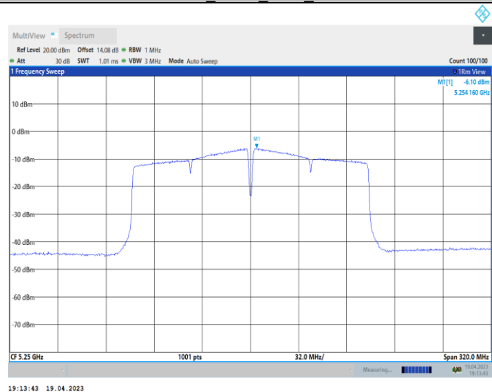
11AC160_Ant10_5250_UNII-2A
