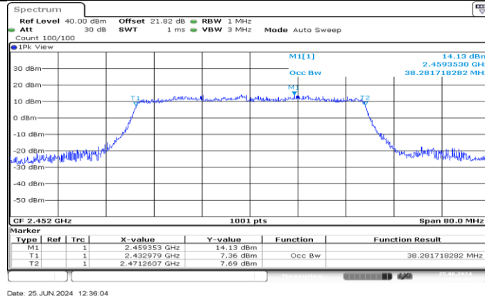
11AX40MIMO_Ant4_2452
