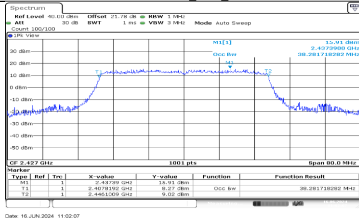
11AX40MIMO_Ant3_2427
