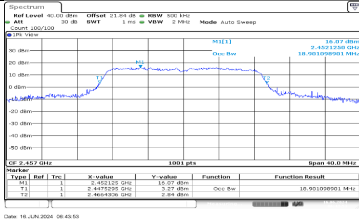
11N20MIMO_Ant3_2457
