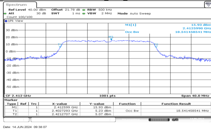
11N20MIMO_Ant3_2412
