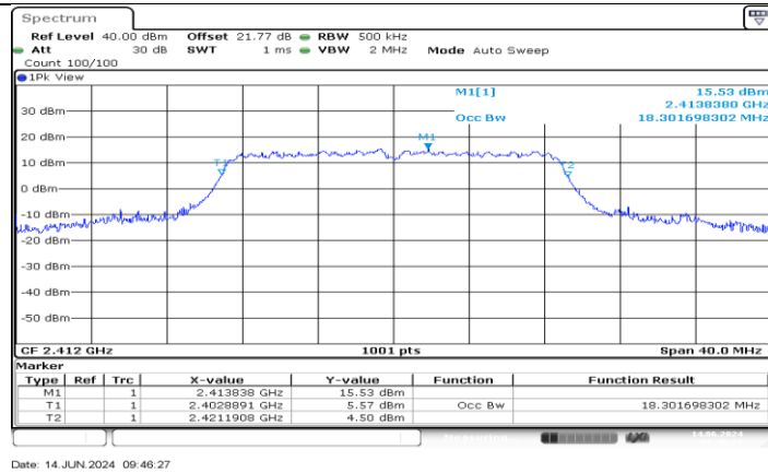
11N20MIMO_Ant4_2412
