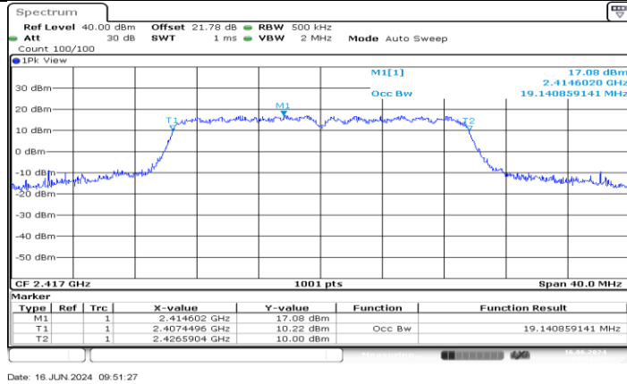
11AX20MIMO_Ant3_2417
