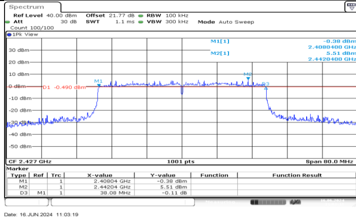
11AX40MIMO_Ant4_2427
