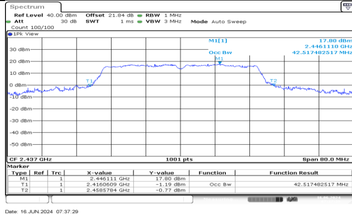
11N40MIMO_Ant4_2437
