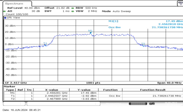
11N20MIMO_Ant4_2457
