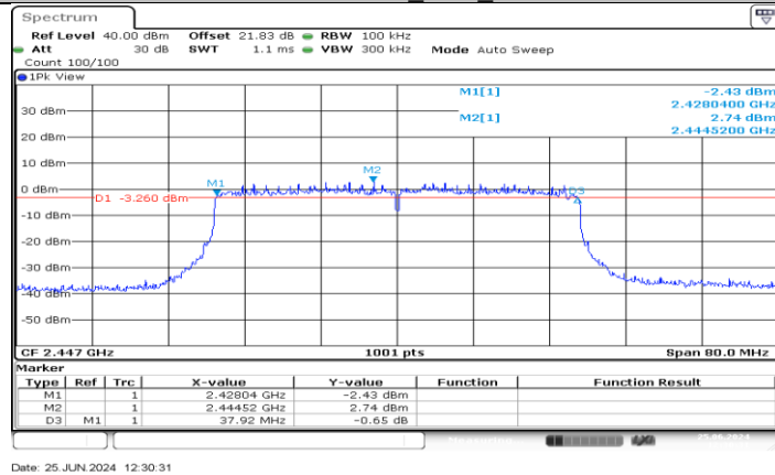
11AX40MIMO_Ant3_2447
