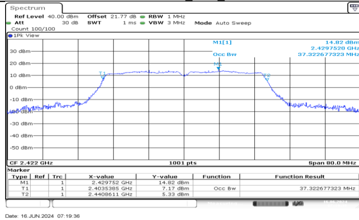
11N40MIMO_Ant4_2422
