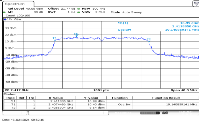
11AX20MIMO_Ant4_2417
