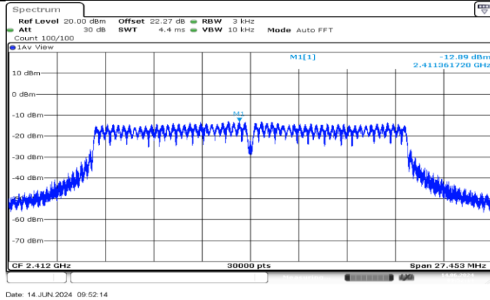
11N20MIMO_Ant4_2412
