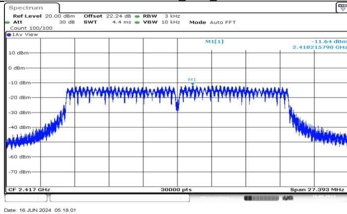
11N20MIMO_Ant3_2417
