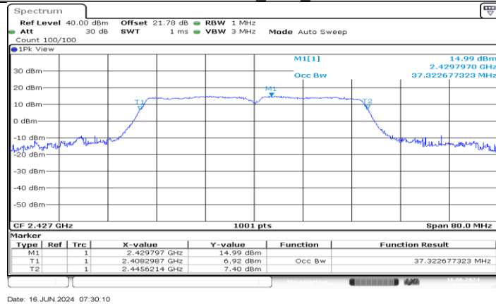
11N40MIMO_Ant3_2427
