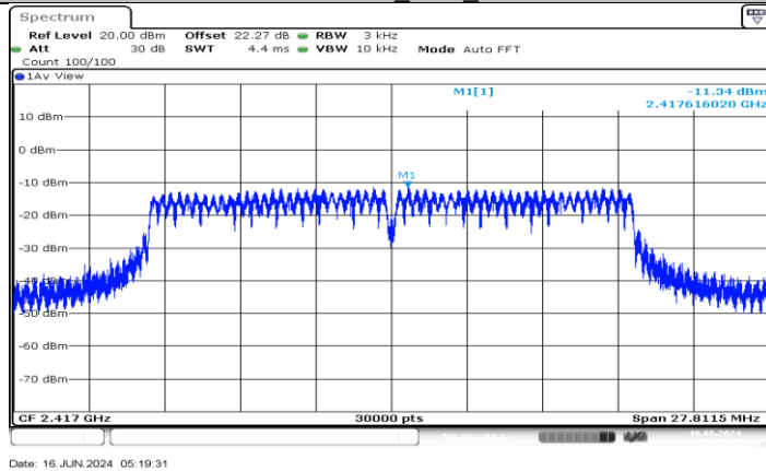
11N20MIMO_Ant4_2417
