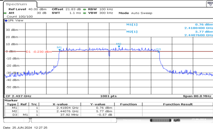
11AX40MIMO_Ant3_2437
