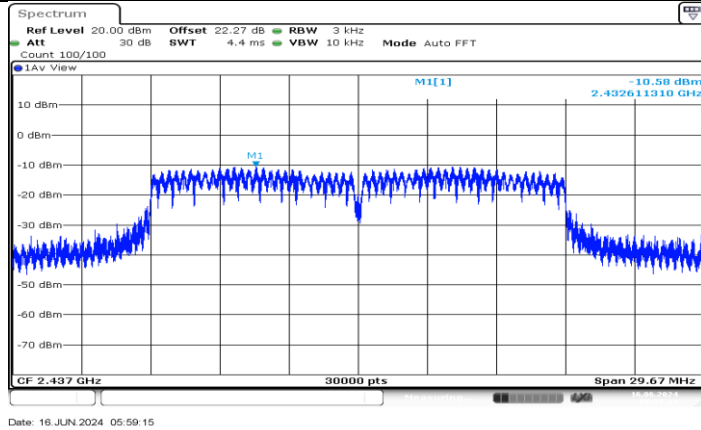
11N20MIMO_Ant4_2437
