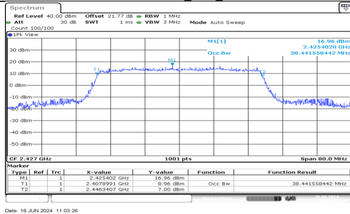
11AX40MIMO_Ant4_2427
