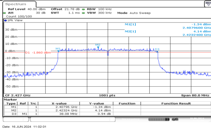
11AX40MIMO_Ant3_2427
