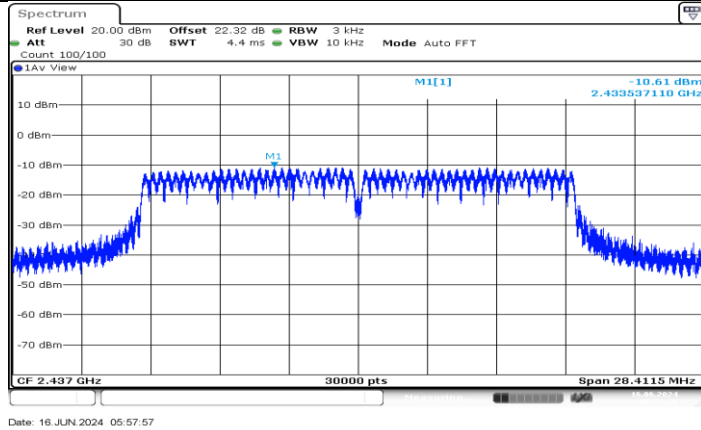
11N20MIMO_Ant3_2437
