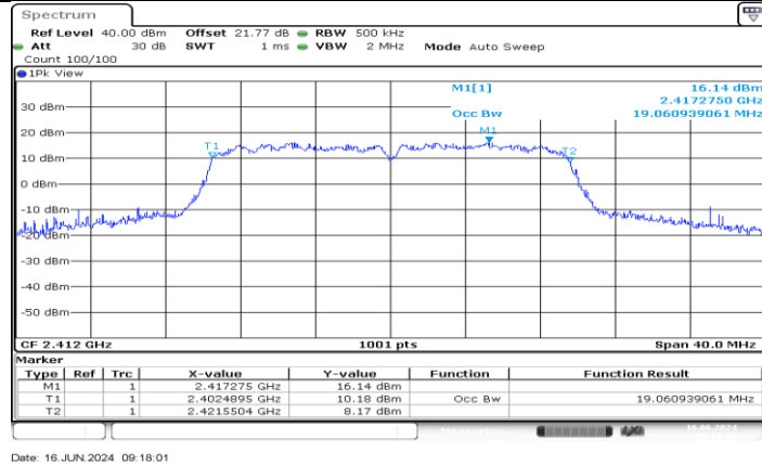
11AX20MIMO_Ant4_2412
