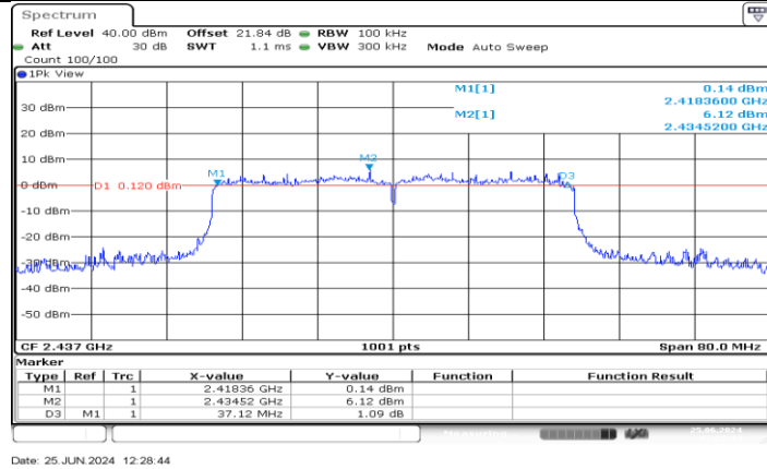
11AX40MIMO_Ant4_2437
