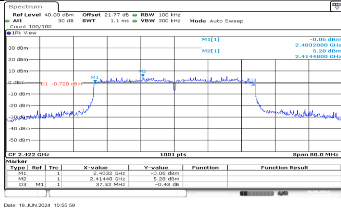
11AX40MIMO_Ant4_2422
