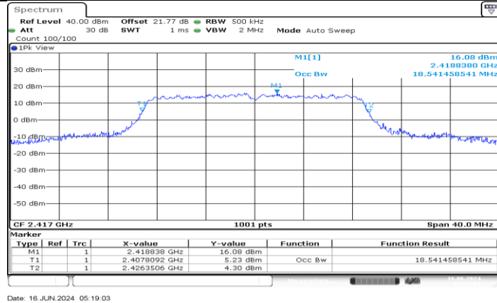
11N20MIMO_Ant4_2417
