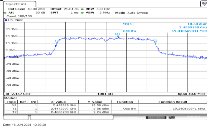
11AX20MIMO_Ant3_2457
