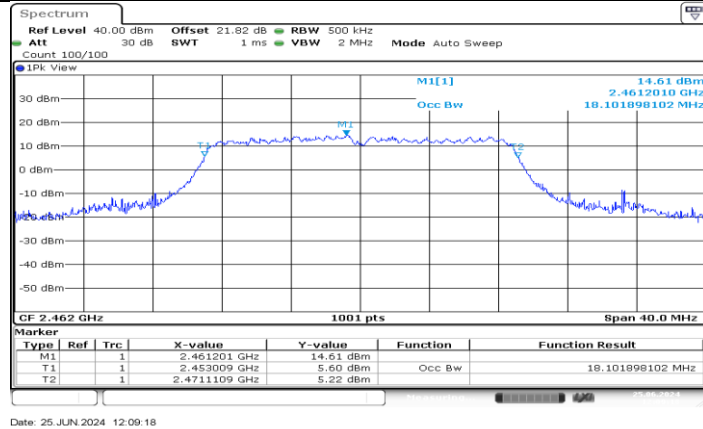
11N20MIMO_Ant4_2462
