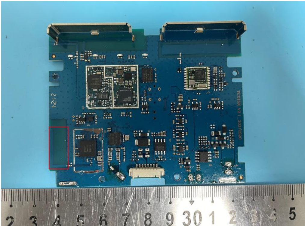
Antenna-NFC
