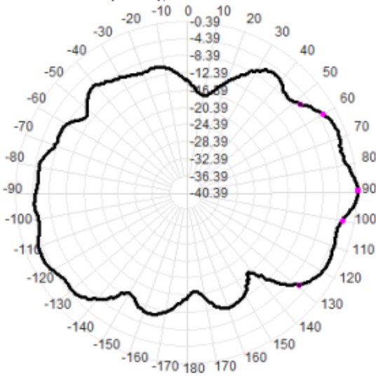
2402.0MHz Total(E2-YZ), Max=-0.39dBi
