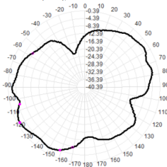
2402.0MHz Total(E1-XZ), Max=-1.81dBi
