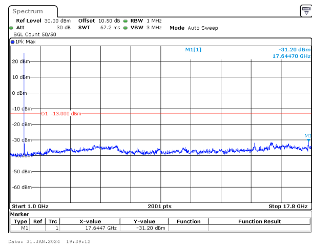
20MHz_15kHz_1770MHz_DFT-s-OFDM QPSK_RB1@0&-31.20 dBm
