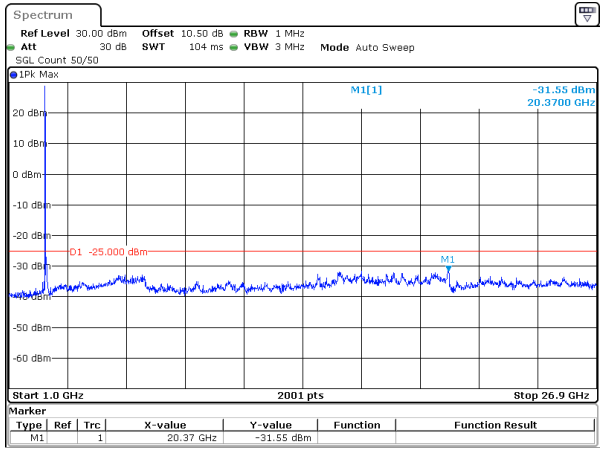
100MHz_30kHz_2640MHz_DFT-s-OFDM QPSK_RB1@0&-31.55 dBm
