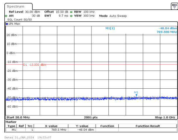
20MHz_15kHz_1720MHz_DFT-s-OFDM QPSK_RB1@0&-48.04 dBm
