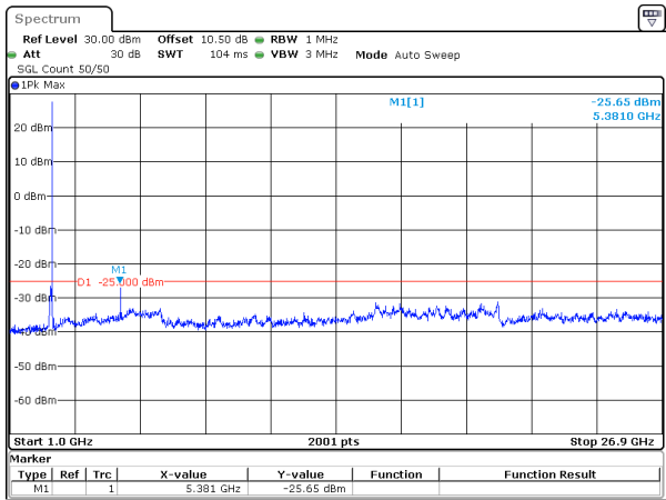
100MHz_30kHz_2640MHz_DFT-s-OFDM QPSK_RB1@272&-25.65 dBm
