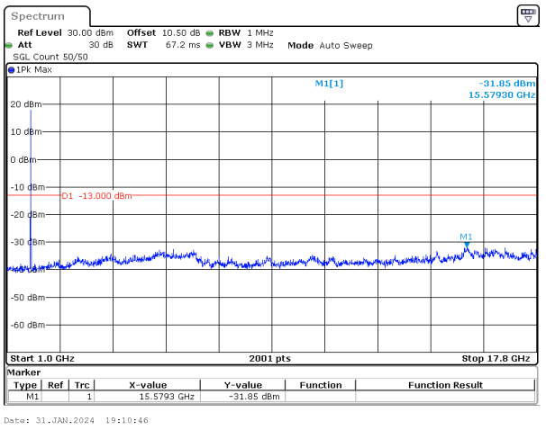
10MHz_15kHz_1745MHz_DFT-s-OFDM QPSK_RB50@0&-31.85 dBm
