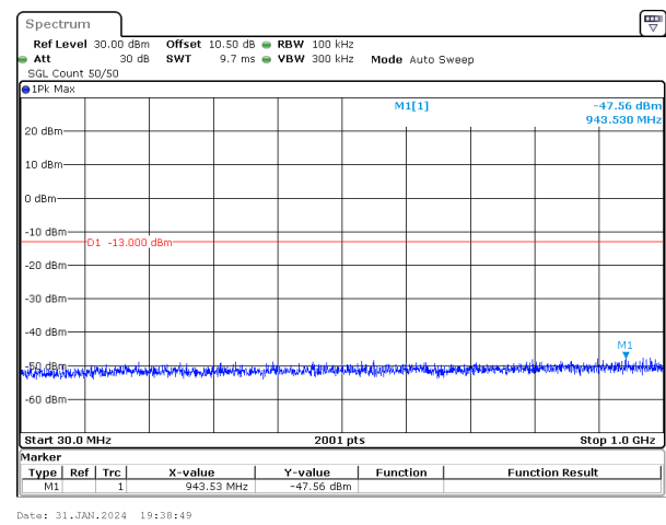
20MHz_15kHz_1770MHz_DFT-s-OFDM QPSK_RB1@0&-47.56 dBm
