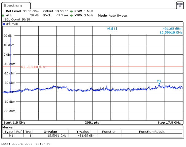
10MHz_15kHz_1775MHz_DFT-s-OFDM QPSK_RB50@0&-31.65 dBm
