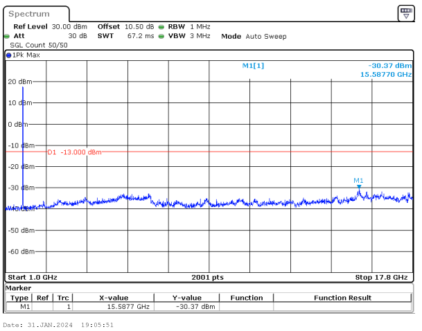
10MHz_15kHz_1715MHz_DFT-s-OFDM QPSK_RB50@0&-30.37 dBm
