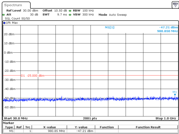
100MHz_30kHz_2640MHz_DFT-s-OFDM QPSK_RB1@272&-47.21 dBm
