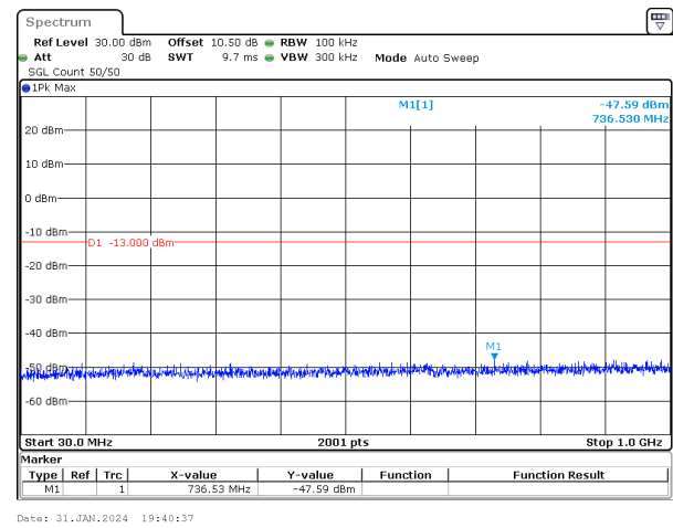
20MHz_15kHz_1770MHz_DFT-s-OFDM QPSK_RB100@0&-47.59 dBm
