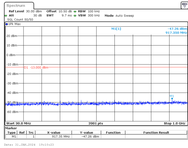
10MHz_15kHz_1745MHz_DFT-s-OFDM QPSK_RB50@0&-47.26 dBm
