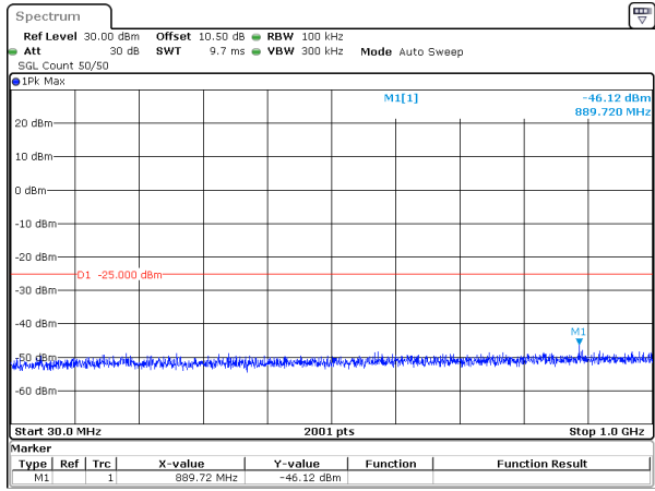
100MHz_30kHz_2640MHz_DFT-s-OFDM QPSK_RB1@0&-46.12 dBm
