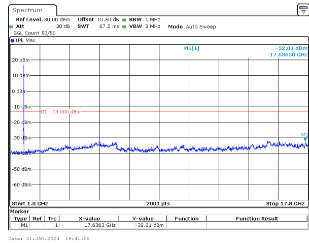
20MHz_15kHz_1770MHz_DFT-s-OFDM QPSK_RB100@0&-32.01 dBm
