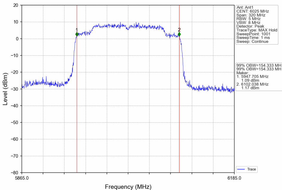
802.11ax(HEW160)_LCH_6025MHz_2xRU996_Left_Ant1_NTNV
