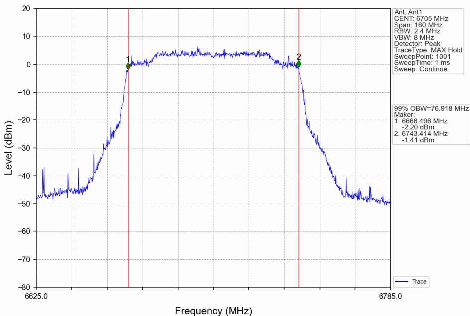
802.11ax(HEW80)_MCH_6705MHz_RU996_Left_Ant1_NTNV
