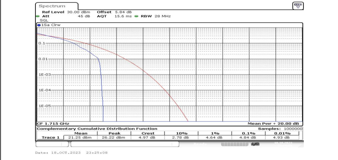
Band4-10MHz-QPSK-20000-1RB#0-PASS
