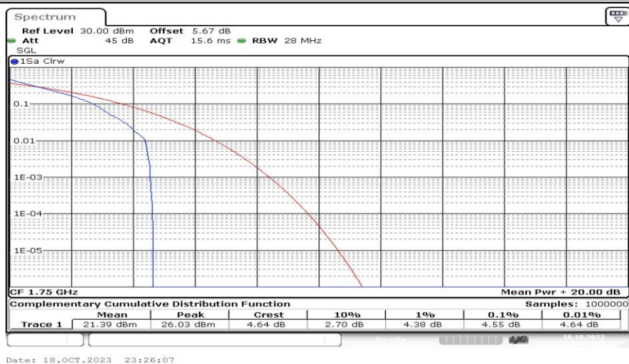
Band4-10MHz-QPSK-20350-1RB#0-PASS
