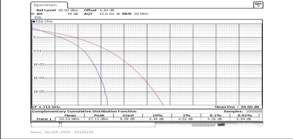
Band4-10MHz-QPSK-20000-50RB#0-PASS
