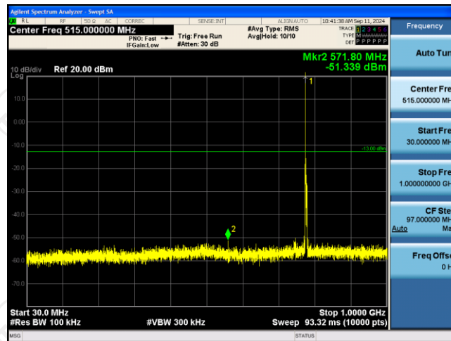
Band13-5MHz-QPSK-23230-1RB#0-Range1:30~1000MHz
