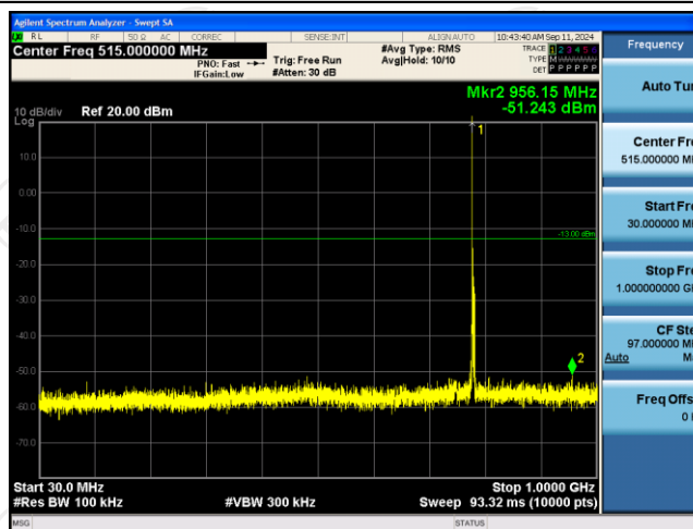
Band13-5MHz-QPSK-23255-1RB#0-Range1:30~1000MHz
