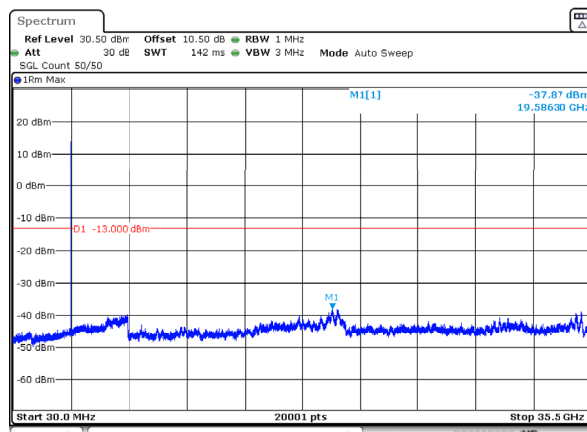
n78_1_10MHz_30kHz_3545MHz_DFT-s-OFDM QPSK_RB1@0 -37.87dBm
