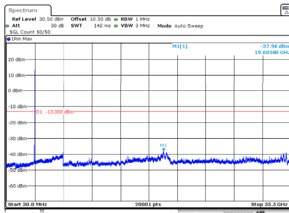
n78_1_30MHz_30kHz_3465MHz_DFT-s-OFDM QPSK_RB1@77 -37.98dBm
