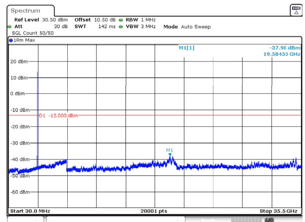
n78_1_40MHz_30kHz_3470MHz_DFT-s-OFDM QPSK_RB1@105 -37.98dBm
