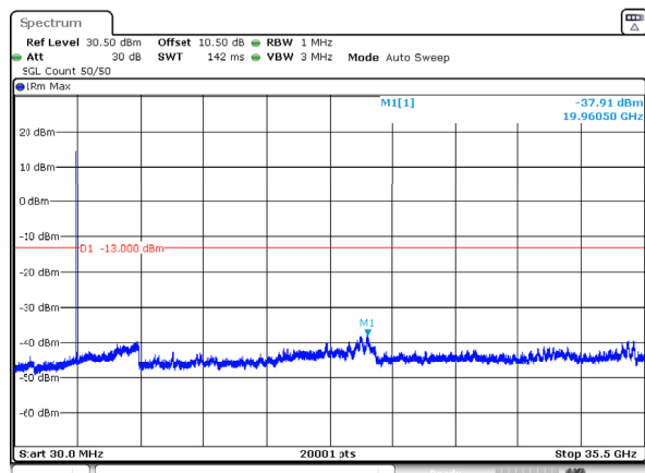
n78_1_20MHz_30kHz_3500MHz_DFT-s-OFDM QPSK_RB1@0 -37.91dBm
