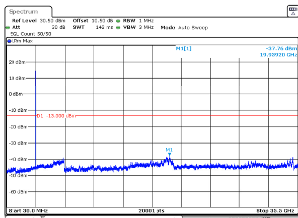
n78_1_10MHz_30kHz_3545MHz_DFT-s-OFDM QPSK_RB1@23 -37.76dBm
