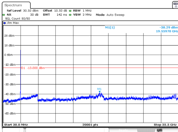
n78_1_30MHz_30kHz_3535MHz_DFT-s-OFDM QPSK_RB75@0 -38.29dBm
