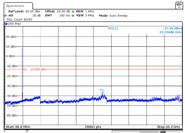
n78_1_10MHz_30kHz_3455MHz_DFT-s-OFDM QPSK_RB24@0 -37.60dBm
