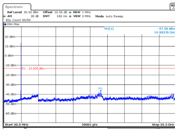
n78_1_60MHz_30kHz_3480MHz_DFT-s-OFDM QPSK_RB1@161 -37.50dBm
