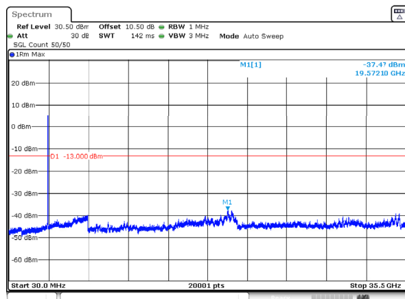
n78_1_20MHz_30kHz_3460MHz_DFT-s-OFDM QPSK_RB50@0 -37.47dBm
