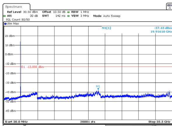
n78_1_50MHz_30kHz_3500MHz_DFT-s-OFDM QPSK_RB1@0 -37.43dBm
