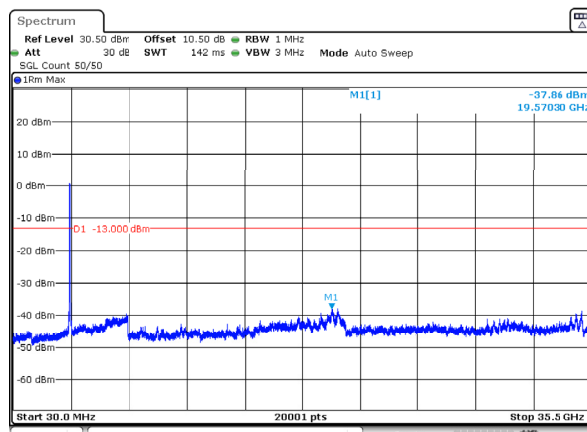
n78_1_60MHz_30kHz_3480MHz_DFT-s-OFDM QPSK_RB162@0 -37.86dBm
