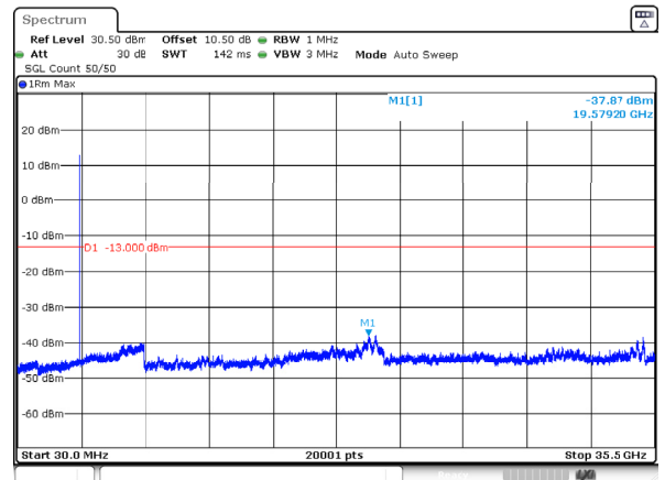
n78_1_10MHz_30kHz_3455MHz_DFT-s-OFDM QPSK_RB1@0 -37.87dBm
