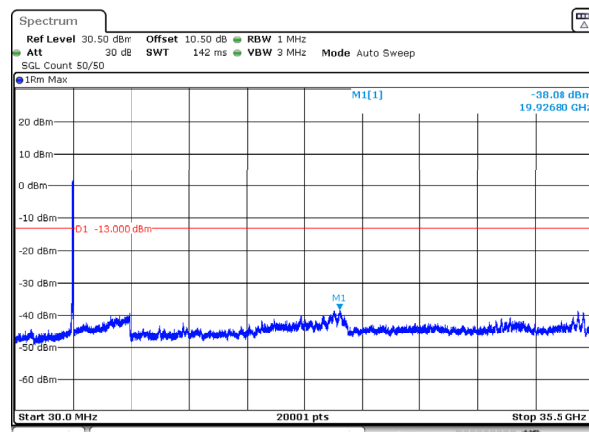
n78_1_50MHz_30kHz_3500MHz_DFT-s-OFDM QPSK_RB128@0 -38.08dBm
