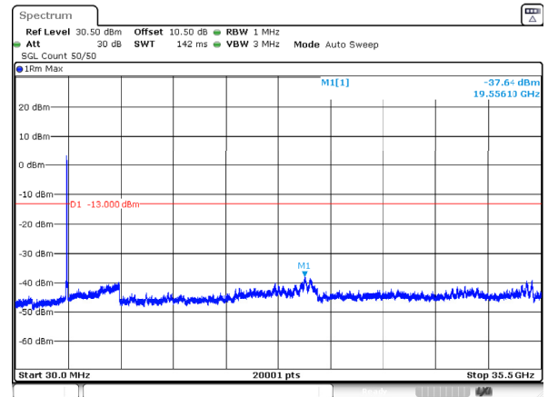
n78_1_40MHz_30kHz_3470MHz_DFT-s-OFDM QPSK_RB100@0 -37.64dBm
