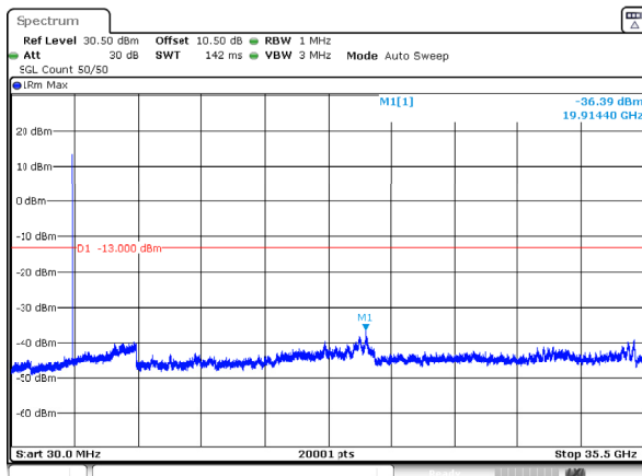
n78_1_10MHz_30kHz_3455MHz_DFT-s-OFDM QPSK_RB1@23 -36.39dBm
