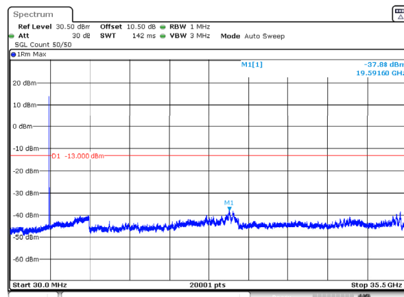
n78_1_50MHz_30kHz_3475MHz_DFT-s-OFDM QPSK_RB1@0 -37.88dBm
