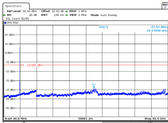
n78_1_15MHz_30kHz_3457.5MHz_DFT-s-OFDM QPSK_RB36@0 -37.91dBm
