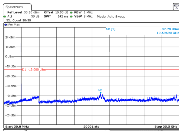
n78_1_60MHz_30kHz_3480MHz_DFT-s-OFDM QPSK_RB1@0 -37.73dBm
