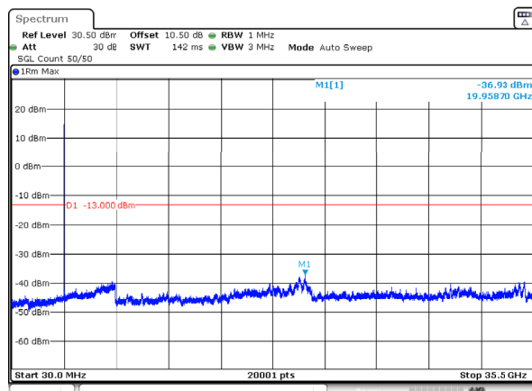
n78_1_15MHz_30kHz_3542.5MHz_DFT-s-OFDM QPSK_RB1@37 -36.93dBm
