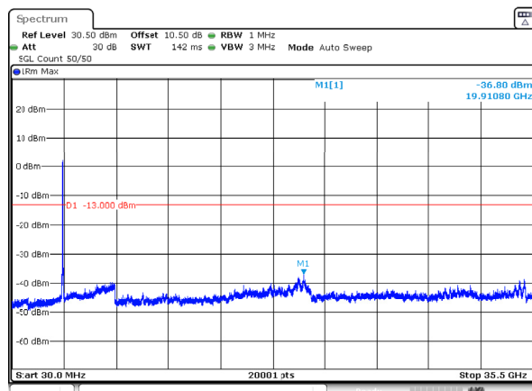
n78_1_50MHz_30kHz_3475MHz_DFT-s-OFDM QPSK_RB128@0 -36.80dBm
