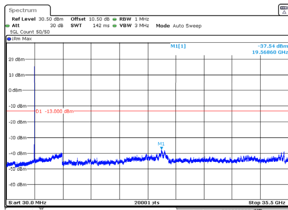
n78_1_50MHz_30kHz_3525MHz_DFT-s-OFDM QPSK_RB1@132 -37.54dBm
