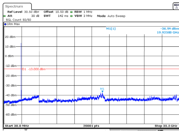
n78_1_20MHz_30kHz_3460MHz_DFT-s-OFDM QPSK_RB1@0 -36.99dBm
