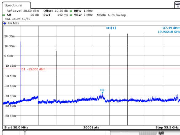
n78_1_30MHz_30kHz_3535MHz_DFT-s-OFDM QPSK_RB1@0 -37.49dBm
