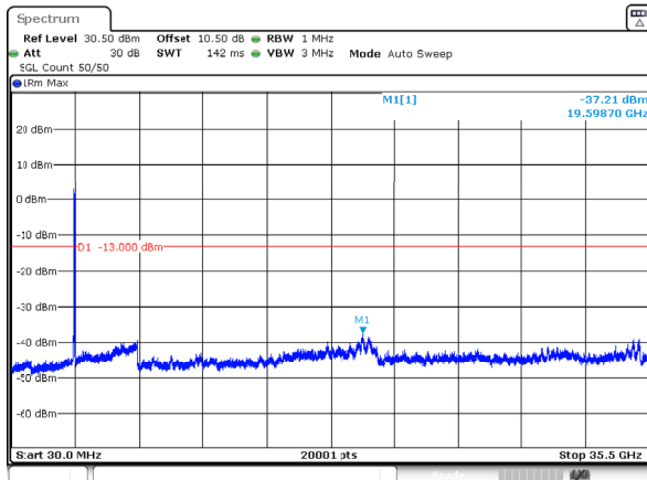
n78_1_40MHz_30kHz_3500MHz_DFT-s-OFDM QPSK_RB100@0 -37.21dBm
