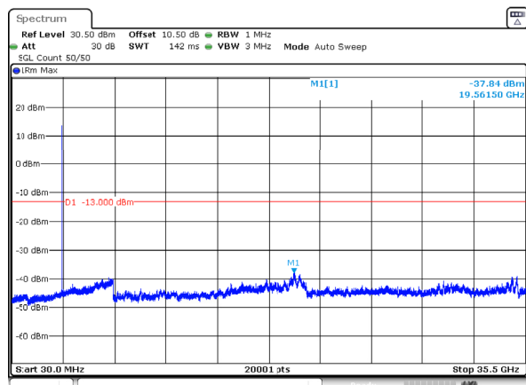
n78_1_10MHz_30kHz_3500MHz_DFT-s-OFDM QPSK_RB1@0 -37.84dBm
