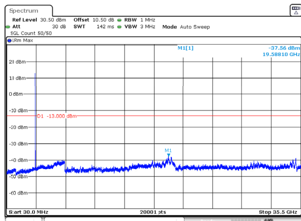
n78_1_30MHz_30kHz_3465MHz_DFT-s-OFDM QPSK_RB1@0 -37.56dBm
