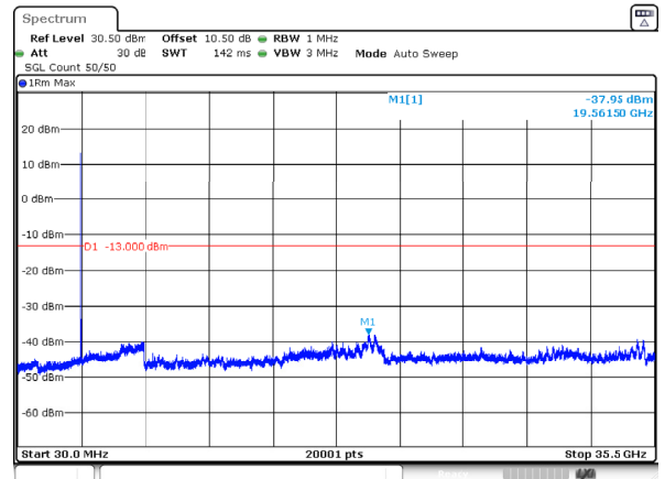
n78_1_40MHz_30kHz_3500MHz_DFT-s-OFDM QPSK_RB1@0 -37.95dBm
