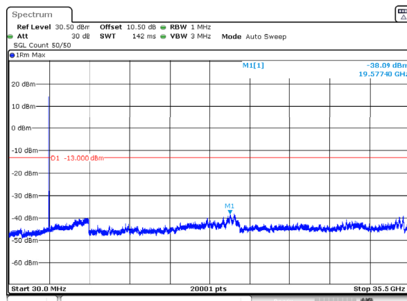
n78_1_50MHz_30kHz_3525MHz_DFT-s-OFDM QPSK_RB1@0 -38.09dBm
