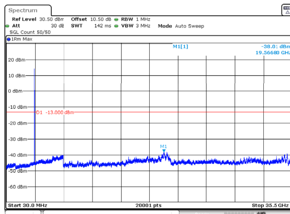
n78_1_15MHz_30kHz_3457.5MHz_DFT-s-OFDM QPSK_RB1@37 -38.01dBm
