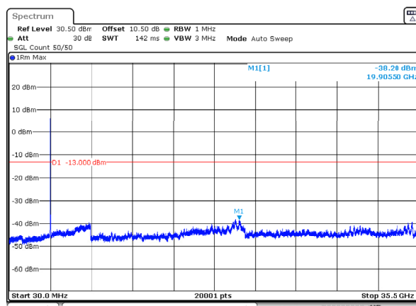
n78_1_20MHz_30kHz_3540MHz_DFT-s-OFDM QPSK_RB50@0 -38.20dBm
