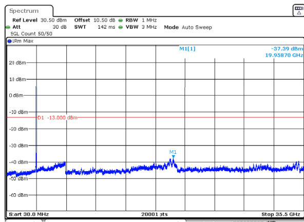
n78_1_20MHz_30kHz_3500MHz_DFT-s-OFDM QPSK_RB50@0 -37.39dBm
