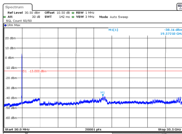
n78_1_30MHz_30kHz_3500MHz_DFT-s-OFDM QPSK_RB75@0 -38.16dBm
