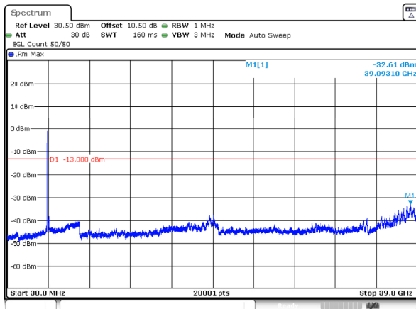
n77_3_100MHz_30kHz_3930MHz_DFT-s-OFDM QPSK_RB270@0 -32.61dBm
