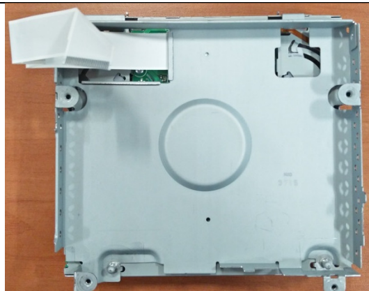
CD BOTTOM
